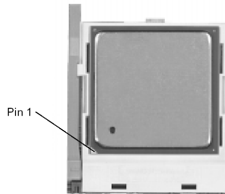
Figura 5. Inserimento della CPU
