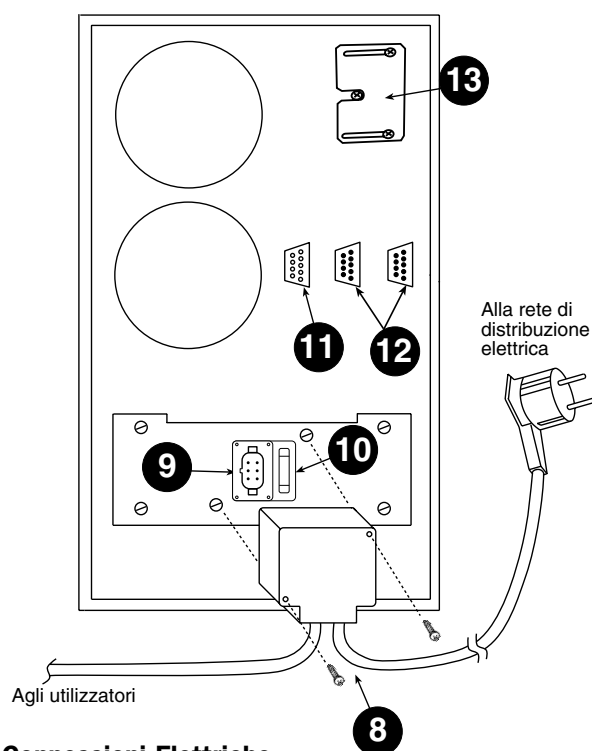
Fig. 2 Connessioni Elettriche
