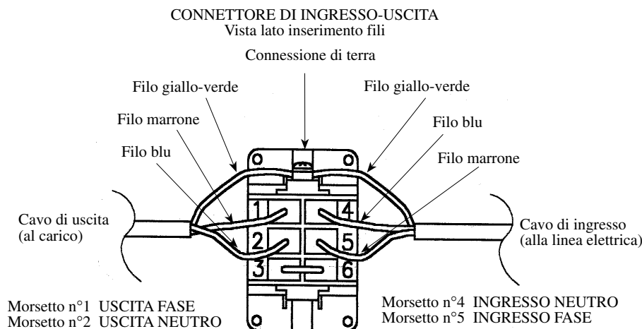
Fig. 4 Morsettiera
