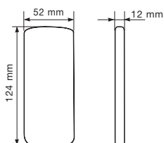
Dimensioni telecomando:
