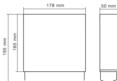
Dimensioni NZ501E:
