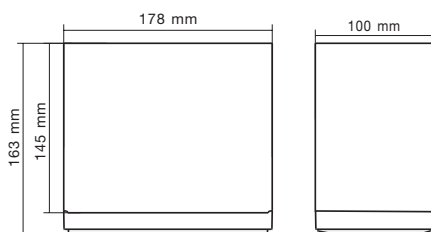
Dimensioni NX501E:
