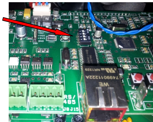
Figura 9 – Dip-Switch di configurazione
