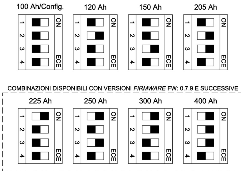
Figura 10 – Configurazione batterie tramite dip-switch
