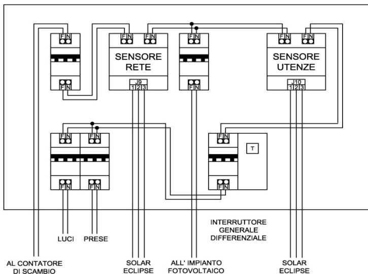
Figura 7 – Schema cablaggio quadro elettrico
