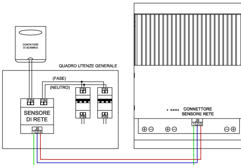
Figura 8 – Cablaggio sensore potenza di rete
