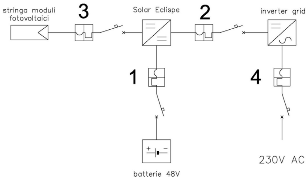
Figura 13 - Schema ordine chiusura/apertura sezionatori avvio/arresto Solar Eclipse
