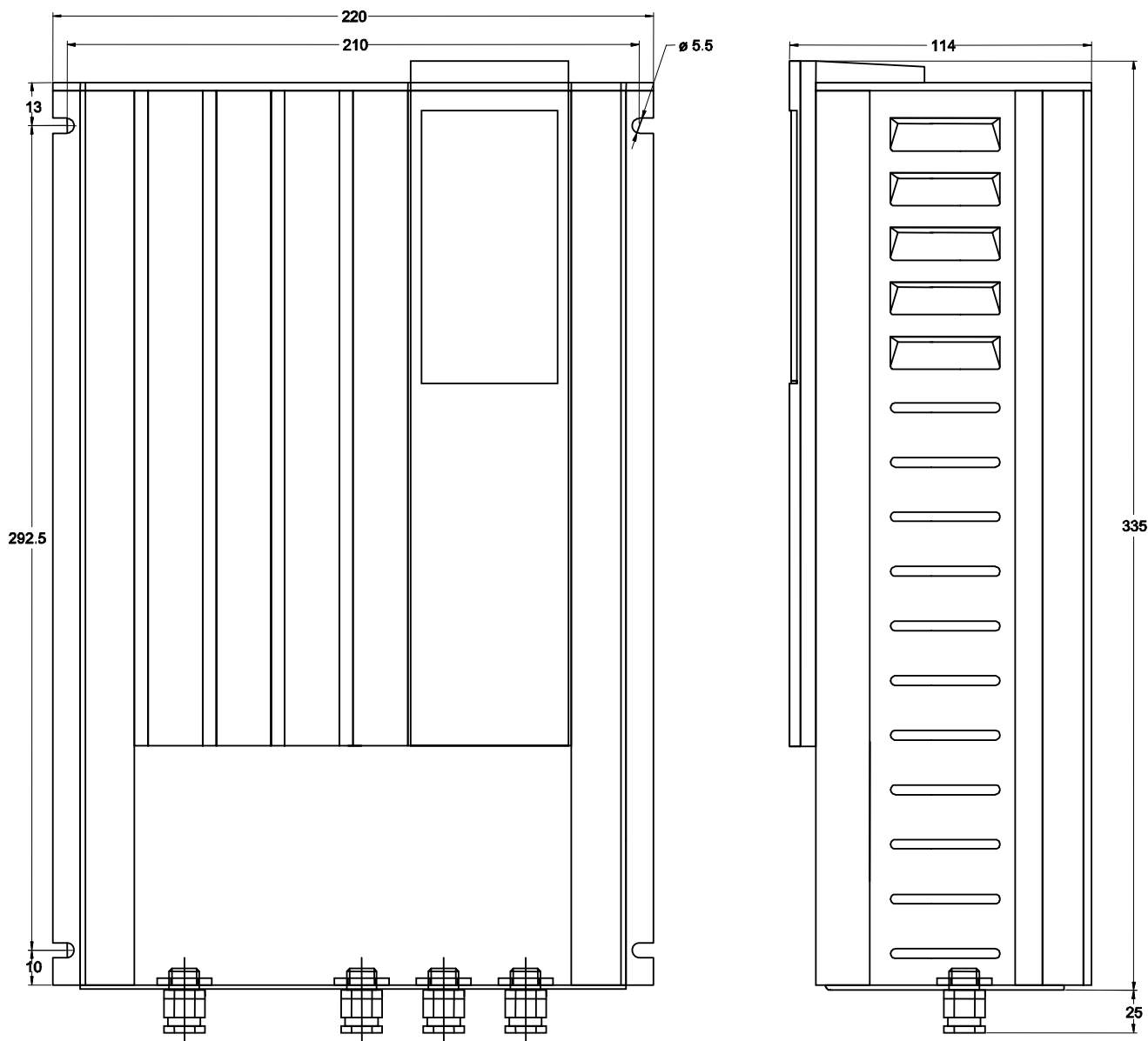
Figura 5: Quote dei Mass Sine 12/800 - 230V e 24/800 - 230V
