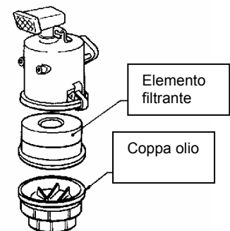
Figura 13 – Filtro aria a bagno d'olio
