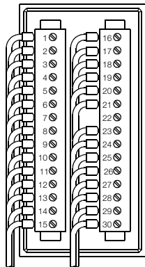
Fig. 2, Disposizione dei contatti
