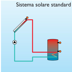
Sistema solare con riscaldamento integrativo
