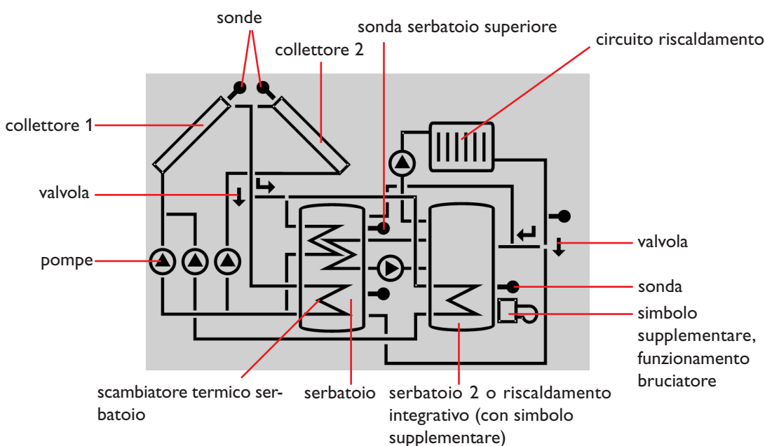
Sonde temperatura
