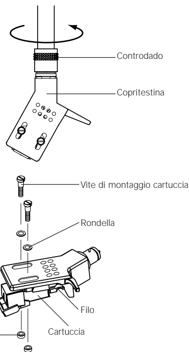
Montaggio parallelo.
