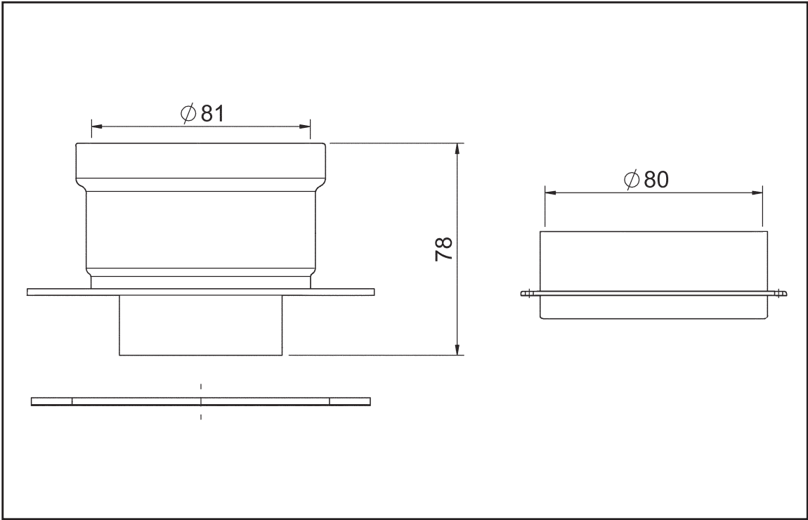
fig. 22 - Accessorio di partenza per condotti separati
