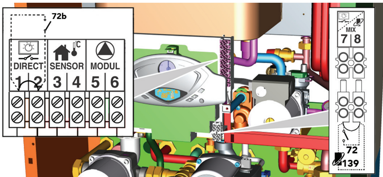
fig. 17 - Accesso alla morsettiera
