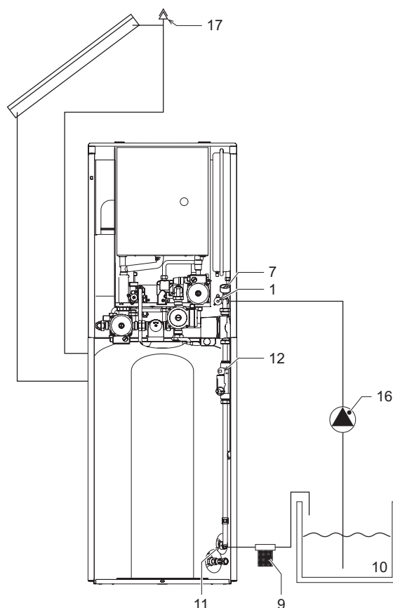
fig. 31 - Circuito solare
