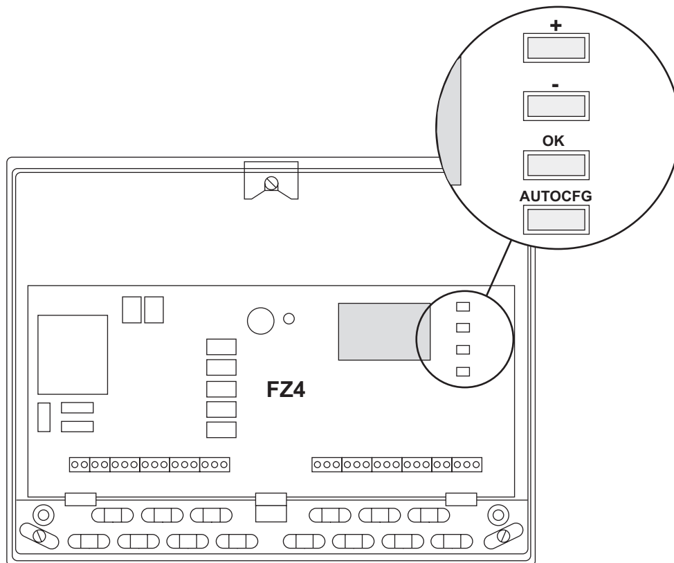
fig. 40 - Centralina FZ4
