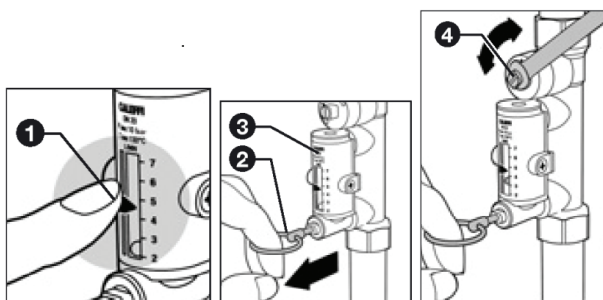
fig. 35 - Limitatore di portata
