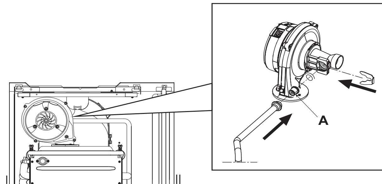
fig. 25 - Sostituzione ugello gas
