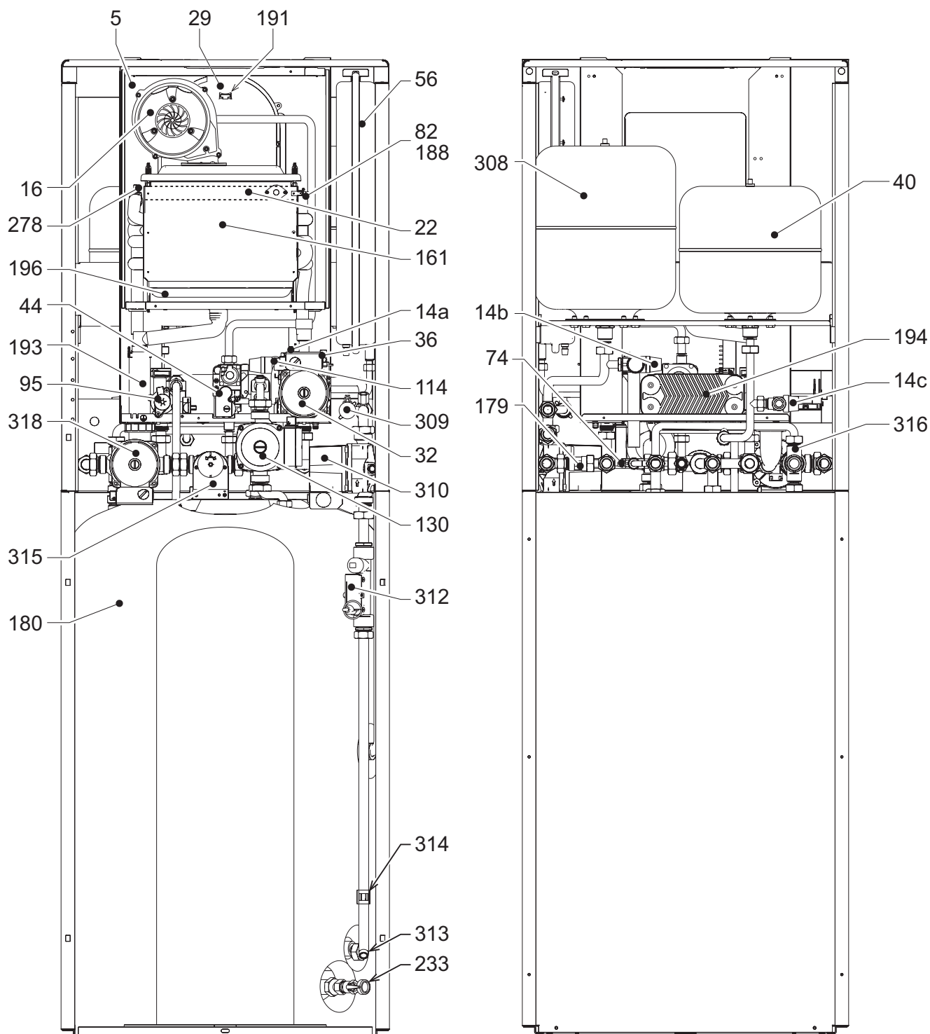
fig. 37 - Componenti principali
