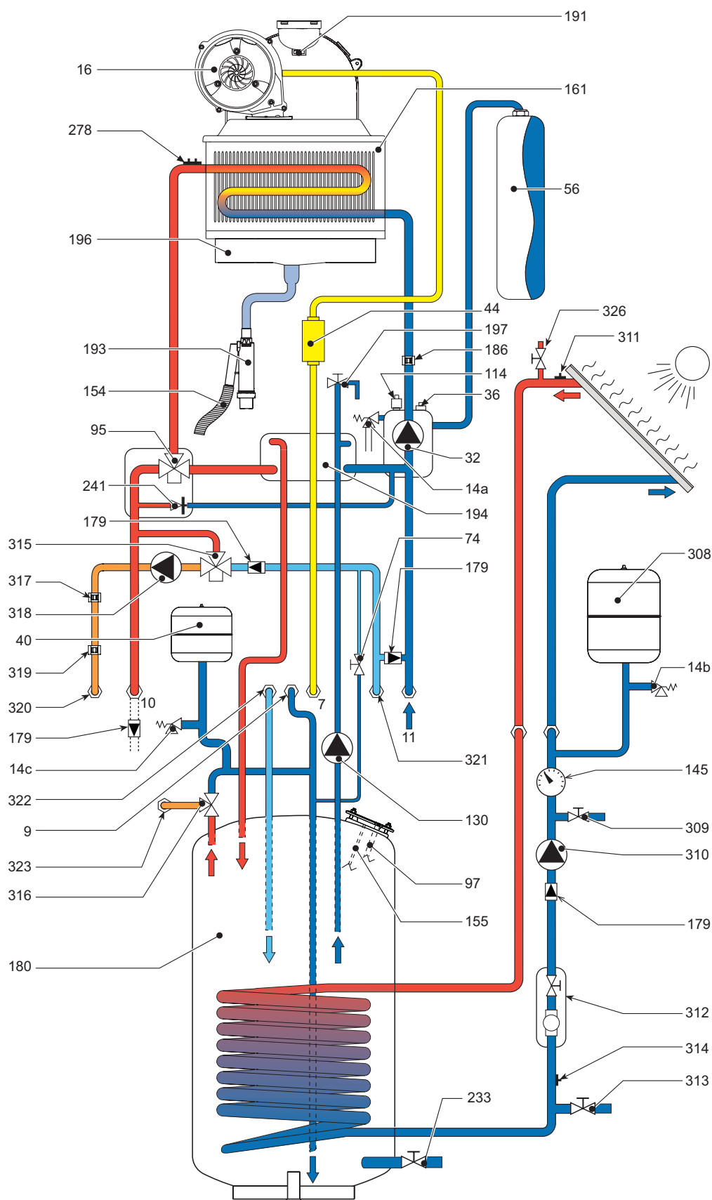
fig. 38 - Circuito idraulico
