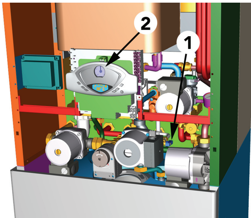
fig. 15 - Rubinetto di caricamento
