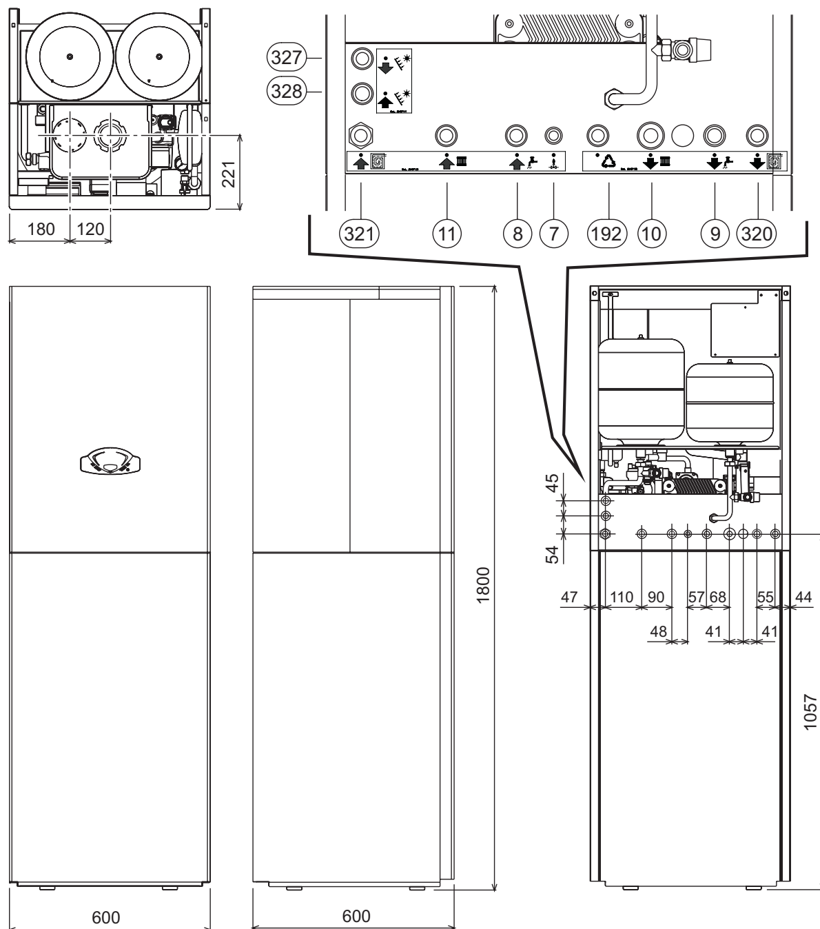
fig. 36 - Dimensioni e attacchi
