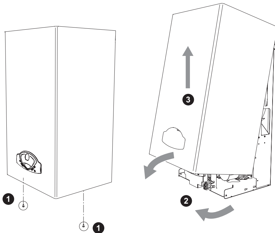
fig. 19 - Apertura del mantello
