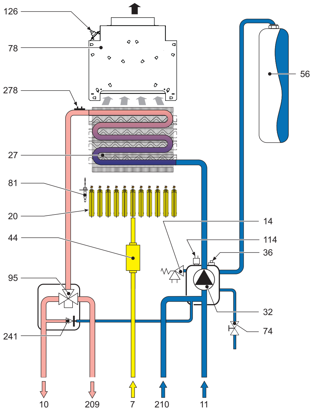
fig. 22 - Circuito idraulico
