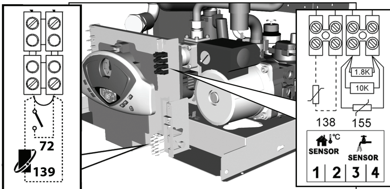
fig. 16 - Accesso alla morsettiere
