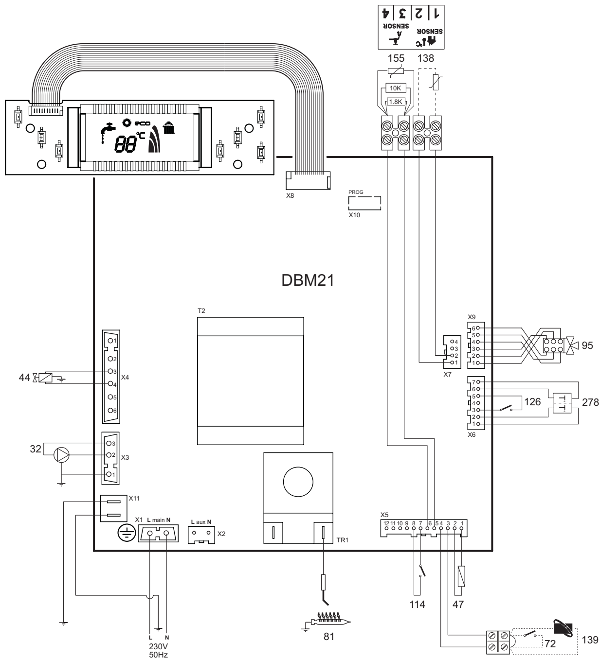
fig. 23 - Schema elettrico
