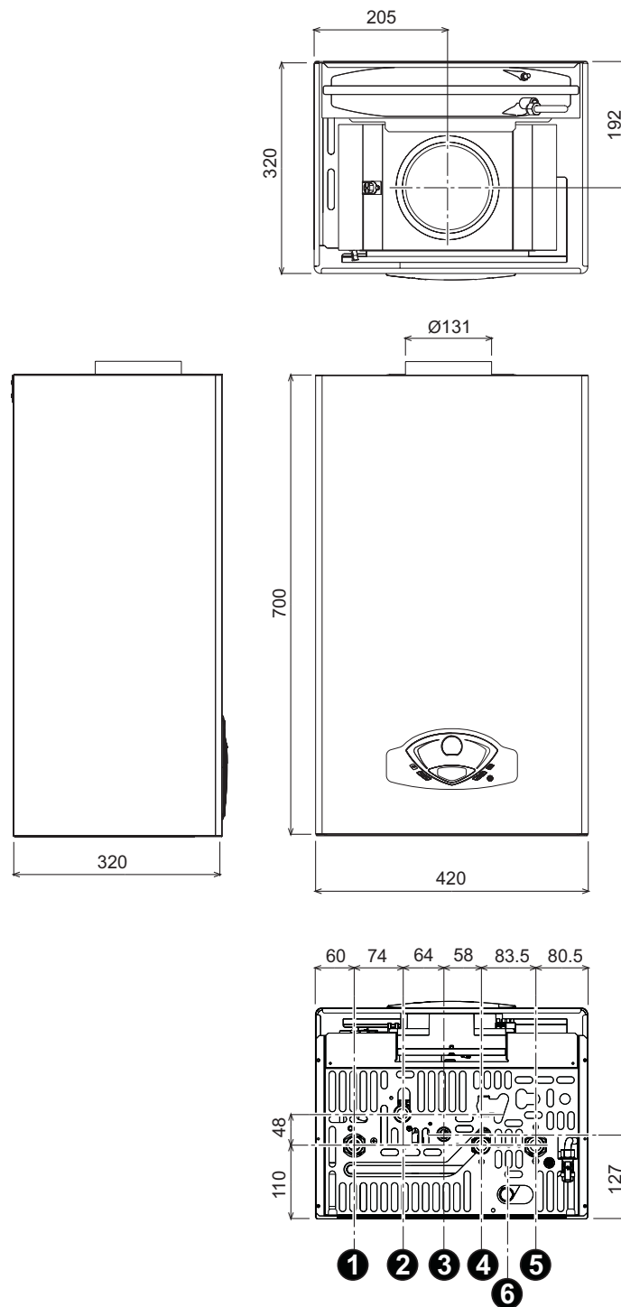
fig. 20 - Dimensioni e attacchi
