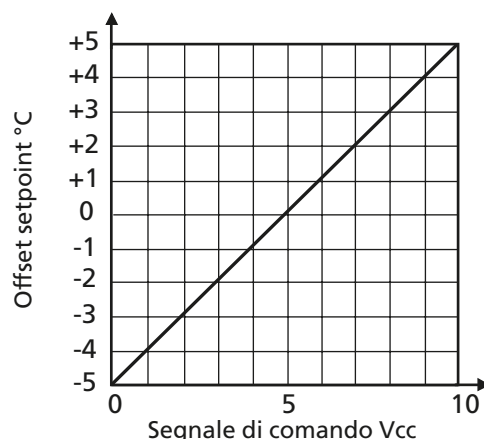
L’offset setpoint determina quanto segue: Segnale di comando 0 Vcc: Il setpoint diminuisce di 5°C. Segnale di comando 5 Vcc: Il setpoint rimane invariato. Segnale di comando 10 Vcc: Il setpoint aumenta di 5°C.
