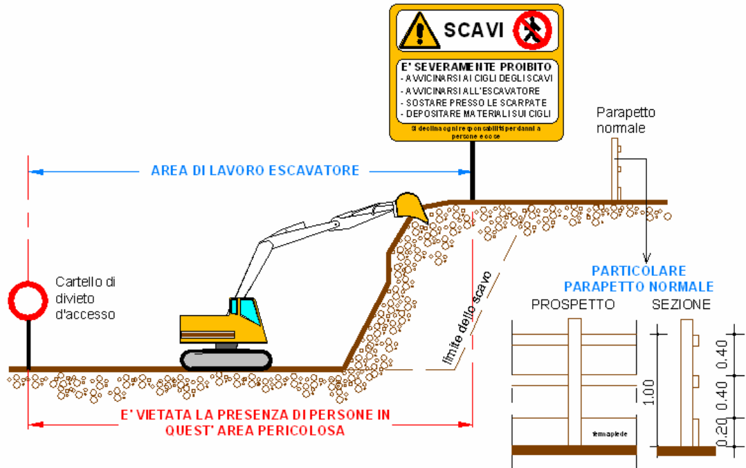
Figura 1 – Organizzazione area di scavo
