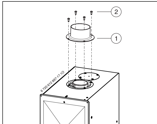
Fig. 17 Fissaggio dell'adattatore per aspirazione aria/ scarico combusti
