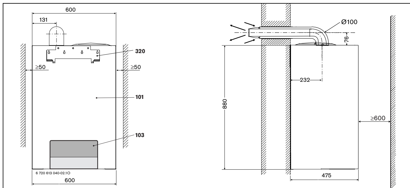
Fig. 2 Logamax U052-24/28T (aspirazione/scarico posteriore)
