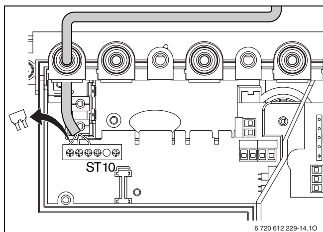
Fig. 19 Allacciamento termostato on/off
