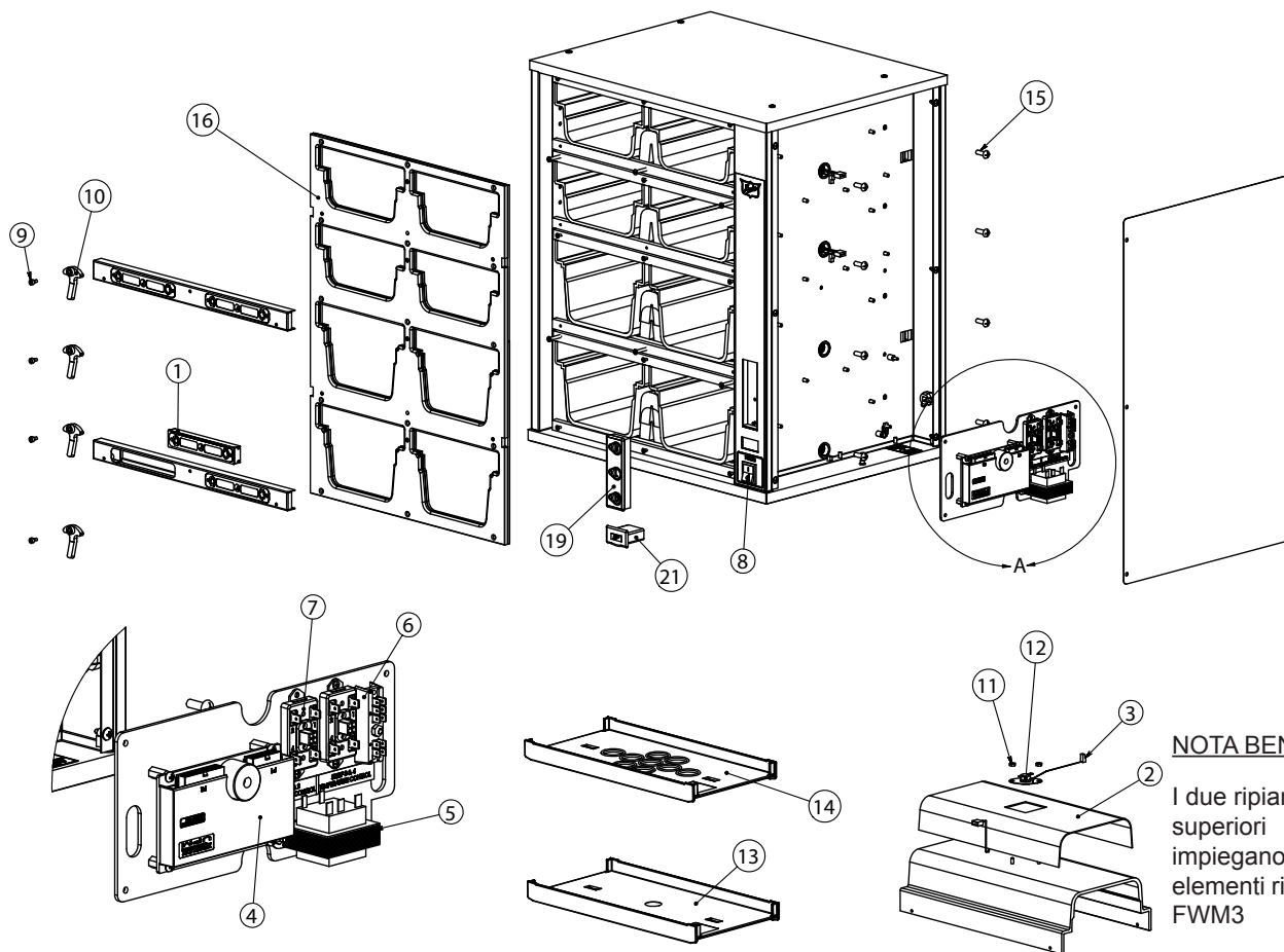
DETTAGLIO A
