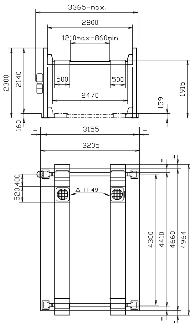
RAV 4401T (Versione ad incasso Recessed version)
