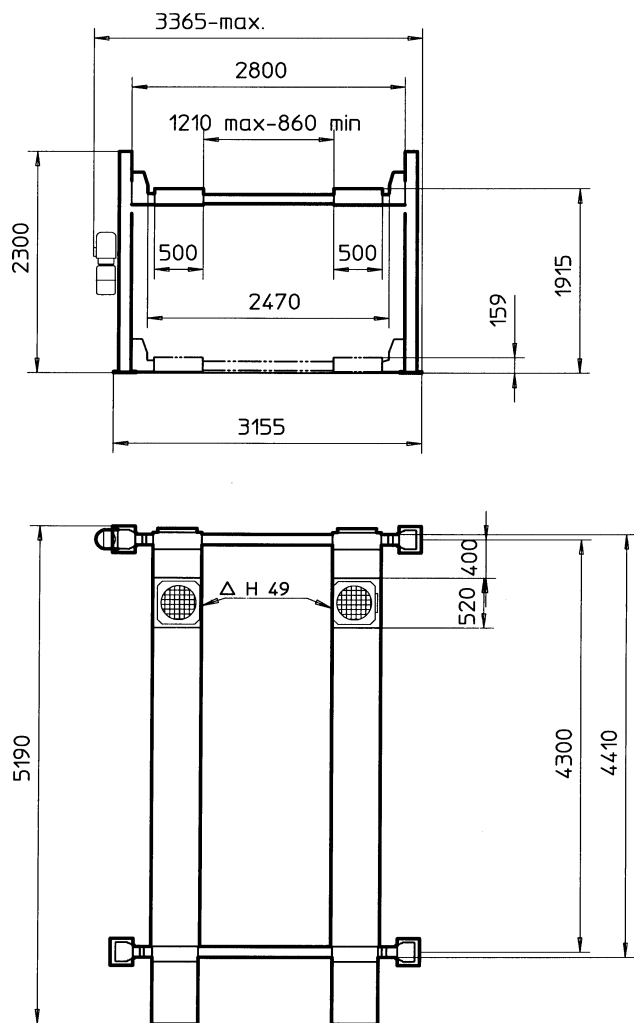
RAV 4401T (Versione a pavimento Floor version)
