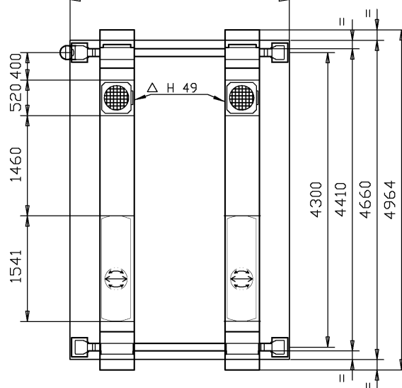
RAV 4402 (Versione ad incasso Recessed version)
