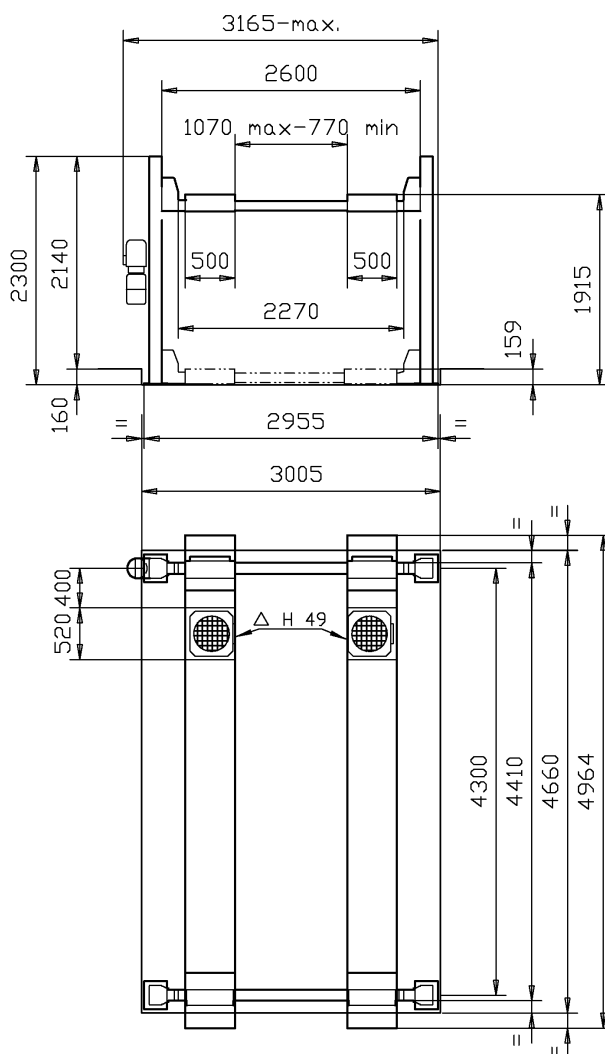
RAV 4351T (Versione ad incasso Recessed version)
