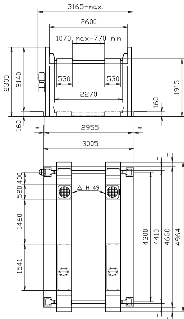
RAV 4352 (Versione ad incasso Recessed version)
