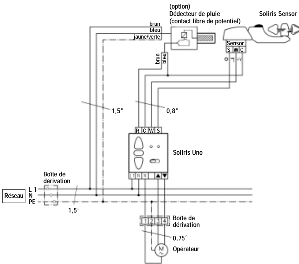
Bornier de branchement
