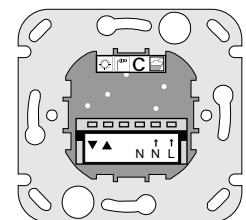
Bornier de branchement
