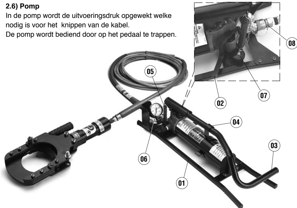
Bild 2 - Onderdelen Pomp
