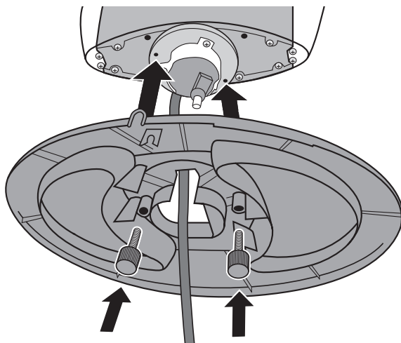
Figure 2 Montage du pied
