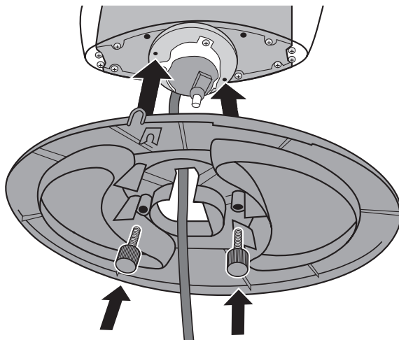
Figuur 2 Voet monteren
