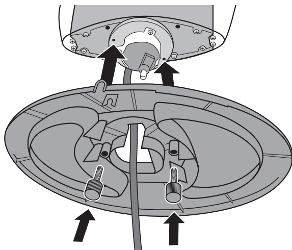
Figura 2 Montaggio della base
