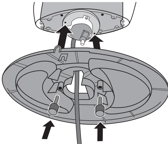
Abbildung 2 Montage des Fußes
