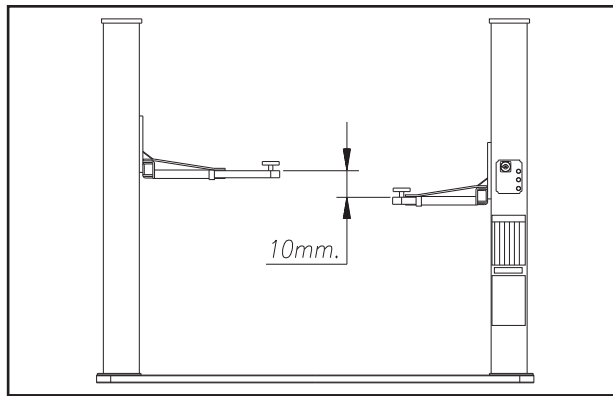
Fig.51 Regolazione dei carrelli
