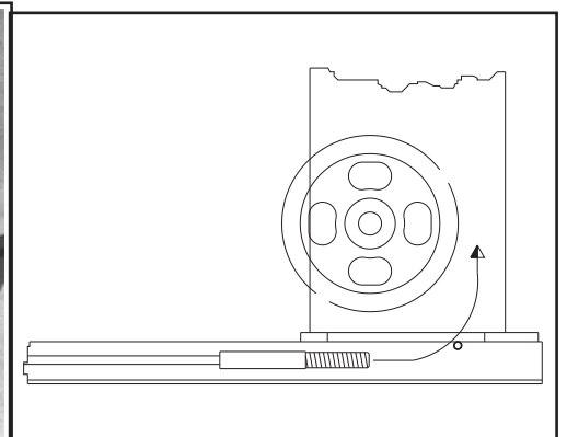
Fig.35 Inserimento del codulo filettato Fig.35 Inserting the threaded end
