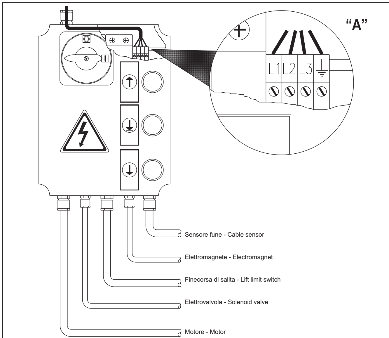
Fig.42 Collegamenti elettrici del quadro
