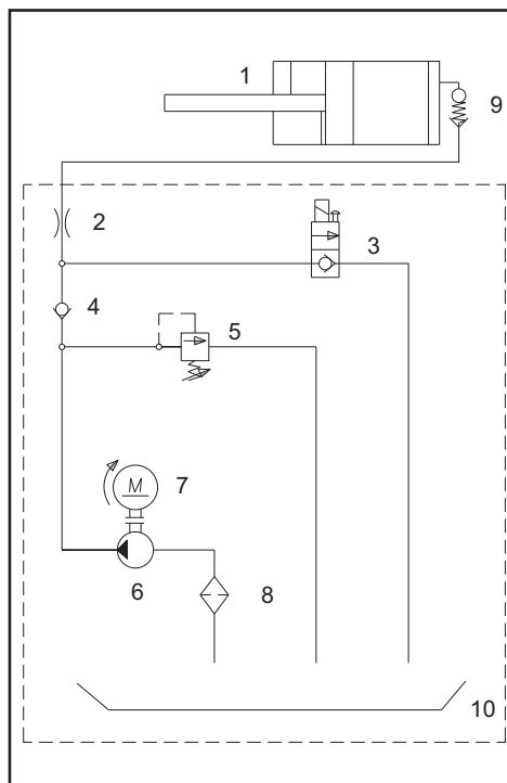
Fig.9 Schema oleodinamico
