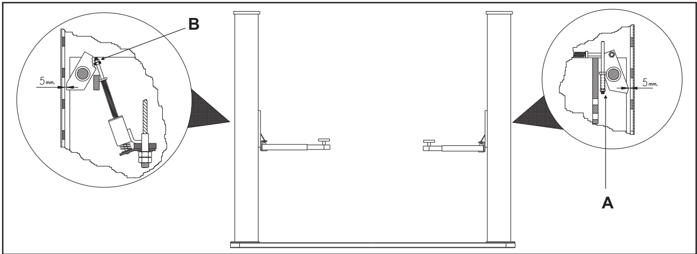
Fig.52 Regolazione dei martelletti
