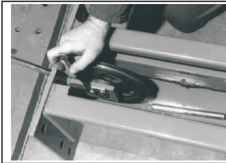
Fig.33 Smontaggio della puleggia Fig.33 Pulley demounting
