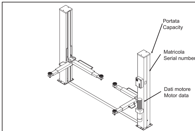
Fig.29 avvisi di sicurezza e targhette applicati sulla macchina.
