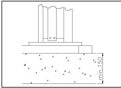
Fig.31 Spessore del pavimento
