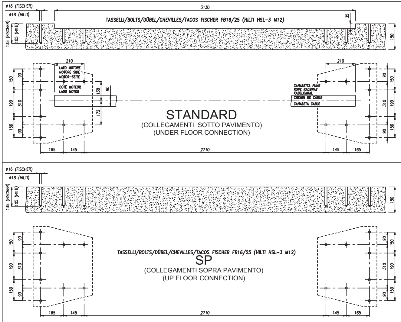
Fig.32 Schema di foratura per fissaggio colonne
