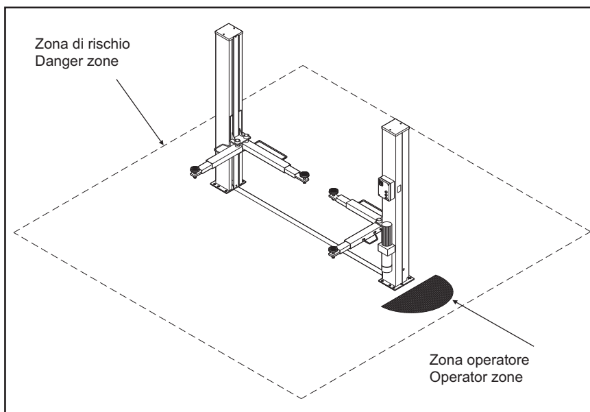
Fig.14 Zone di lavoro
