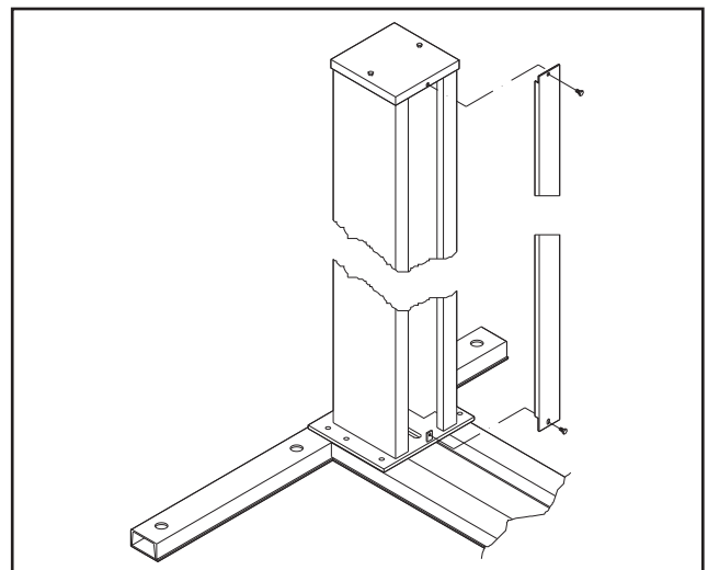
Fig.60 Montaggio dei carter Fig.60 Casing assembly
