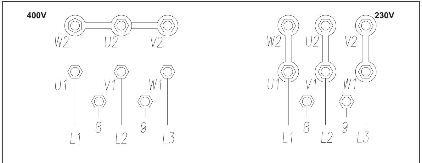
Fig.43 Collegamenti motore e trasformatore
