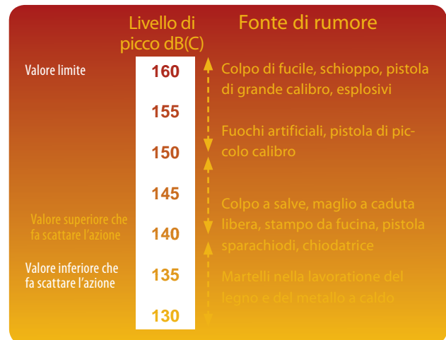
Figura 2.3 Livelli di pressione acustica di picco tipici delle fonti impulsive
