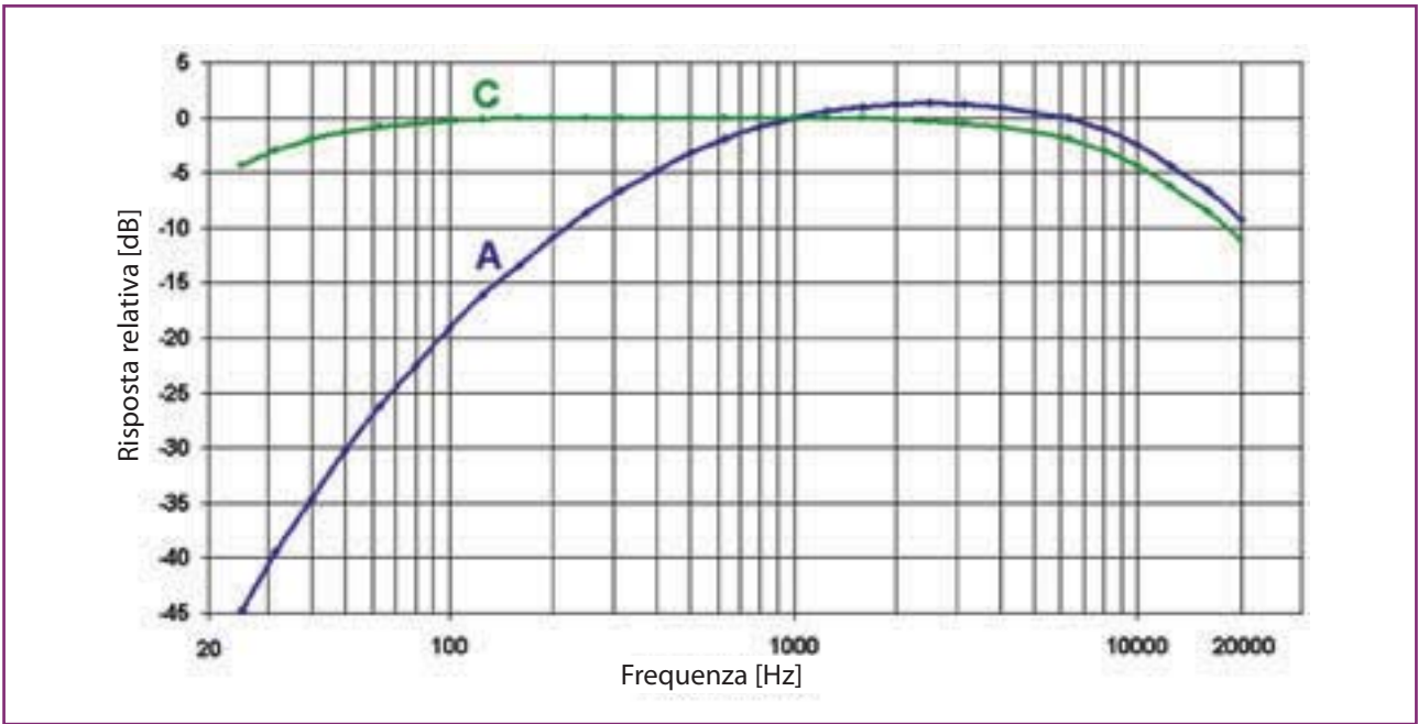
Figura 1.21 - Curve di ponderazione
