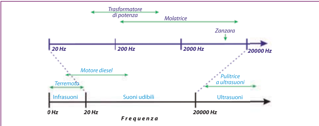
Figura 1.8 Intervalli sonori sulla scala della frequenza
