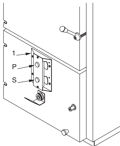
1 Gruppo regolazione aria S Viti di regolazione aria secondaria P Vite di regolazione aria primaria
