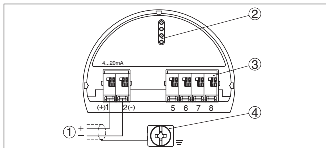
Figura 10: Vano dell'elettronica e di connessione della custodia ad una camera
