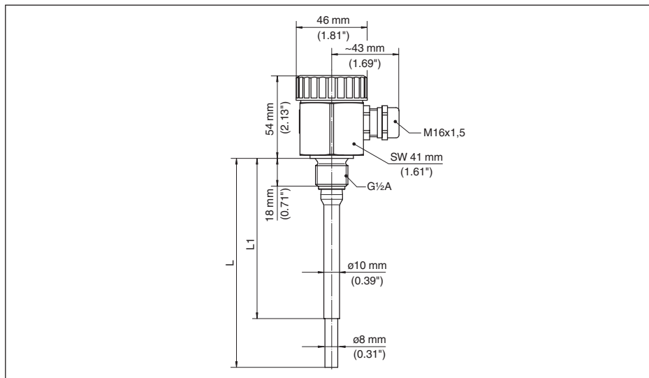
Figura 9: Sonda conduttiva a barra EL 1
