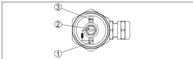
Figura 6: Vano di connessione
