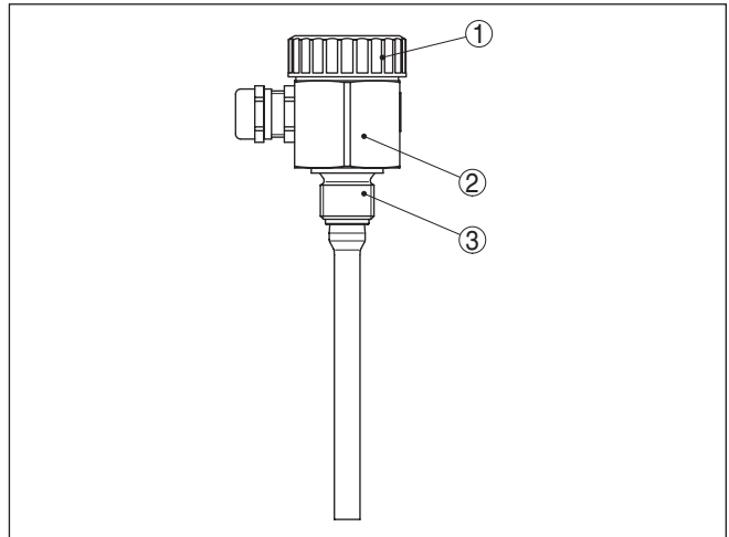
Figura 1: Sonda conduttiva a barra EL 1
