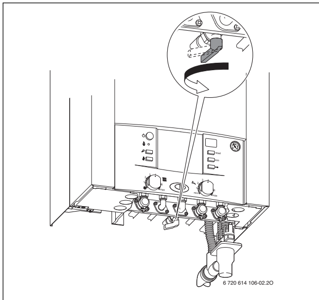
Fig. 3 Vista caldaia con placca rubinetteria, accessorio DOS GA 5/18
