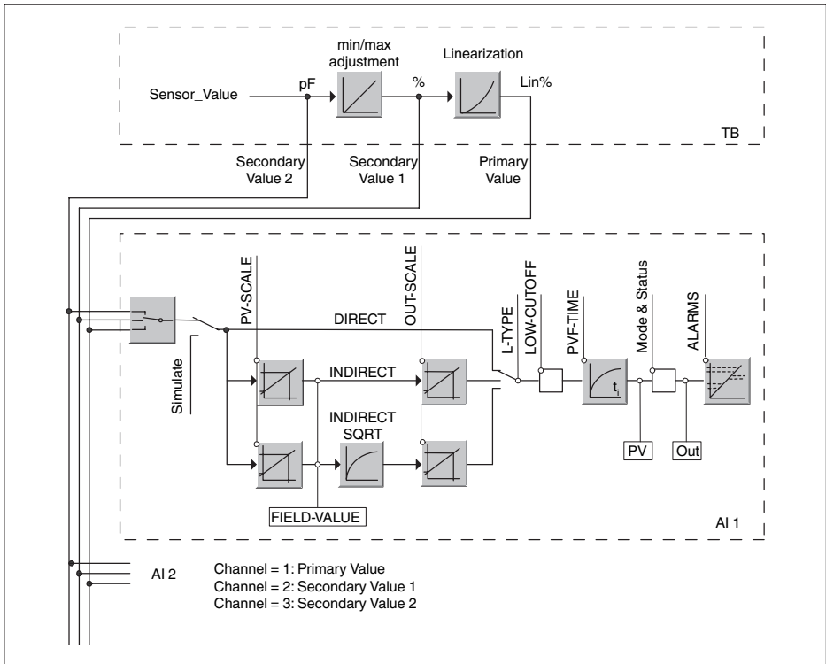
Figura 21: Elaborazione valore di misura VEGACAL 67
