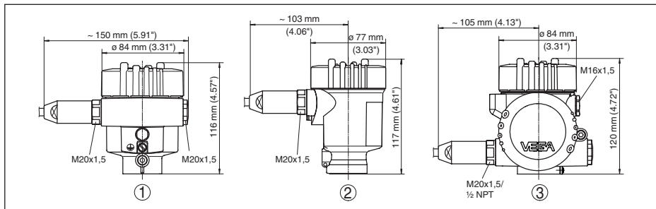
Figura 24: Le differenti custodie con grado di protezione IP 66/IP 68 (1 bar) - con tastierino di taratura con display incorporato l'altezza della custodia aumenta di 9 mm/0.35 in
