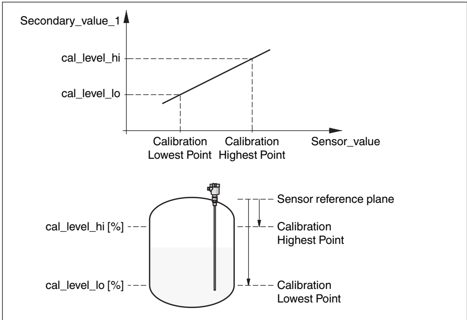
Figura 22: Taratura VEGACAL 67
