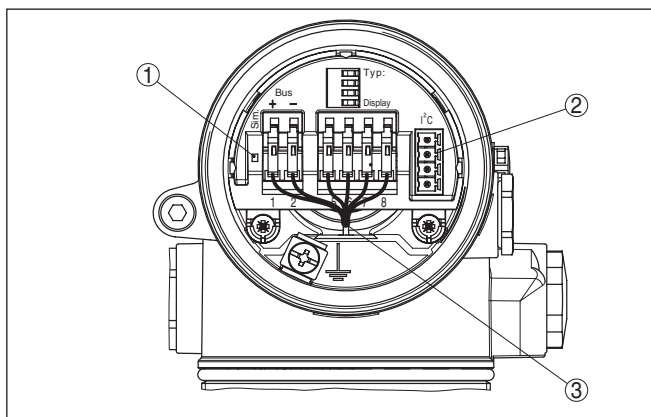
Figura 11: Vano dell'elettronica con custodia a due camere
