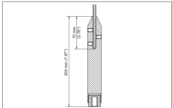
Figura 19: Tenete conto del peso tenditore ed accorciate la fune in proporzione.
