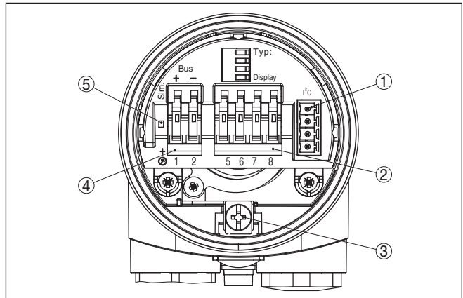
Figura 8: Vano dell'elettronica e di connessione della custodia ad una camera
