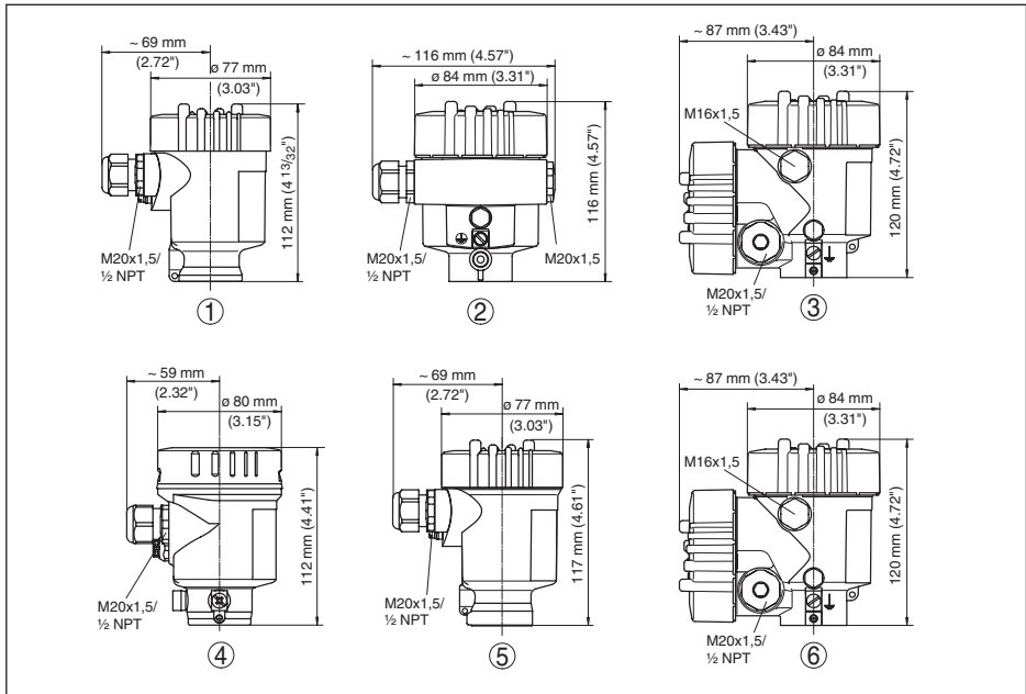
Figura 23: Le differenti custodie con grado di protezione IP 66/IP 68 (0,2 bar) - con tastierino di taratura con display incorporato l'altezza della custodia aumenta di 9 mm/0.35 in
