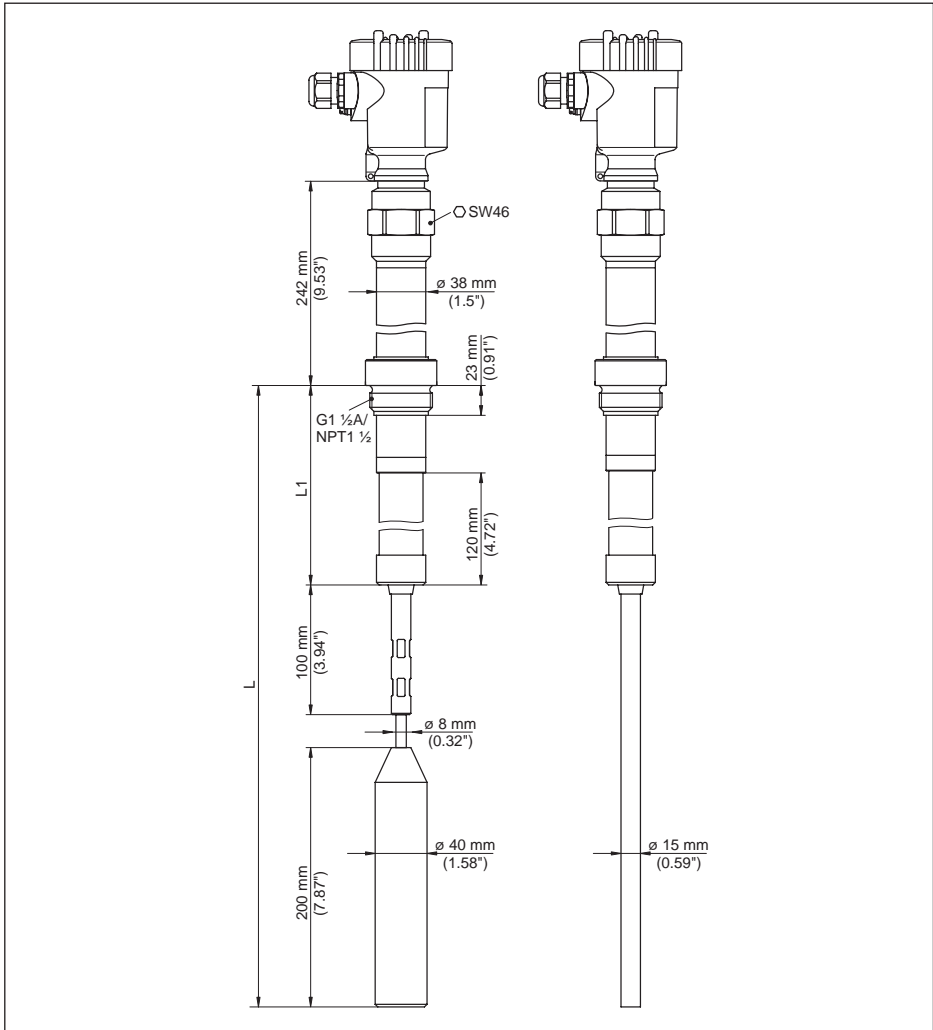
Figura 25: VEGACAL 67, esecuzione filettata G1½ A (ISO 228 T1) e 1½ NPT, -50 ... +300 °C (-58 ... +572 °F)
