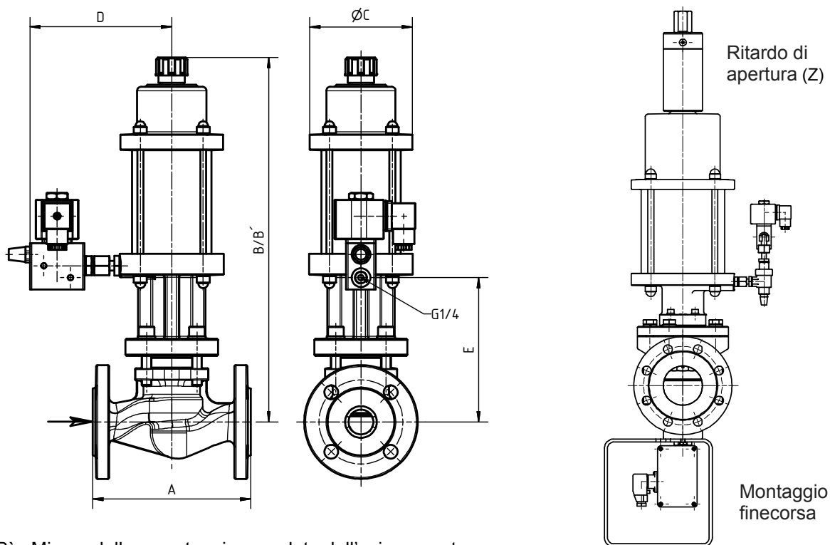
speciale ...-EPVA...(N)H.-4.Z.. + Montaggio finecorsa
