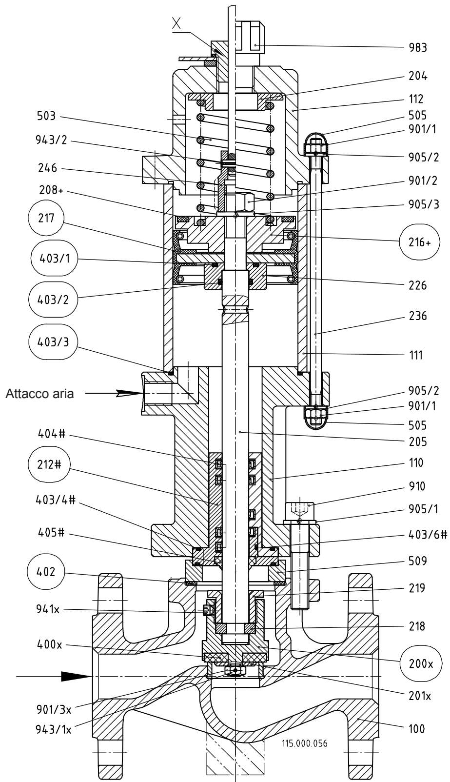
Fig. 2 Disegno in sezione 6-4-EPVA...N(H).. DN15 – DN25; 3-4-EPVA 15N(H)..; 6-4-EPVA 15N(H)..; 6-4-EPVA 20N..
