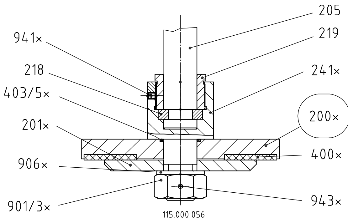
Fig. 3 Testa della valvola da DN 80
