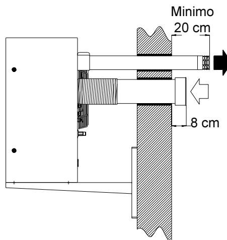
Vista laterale
