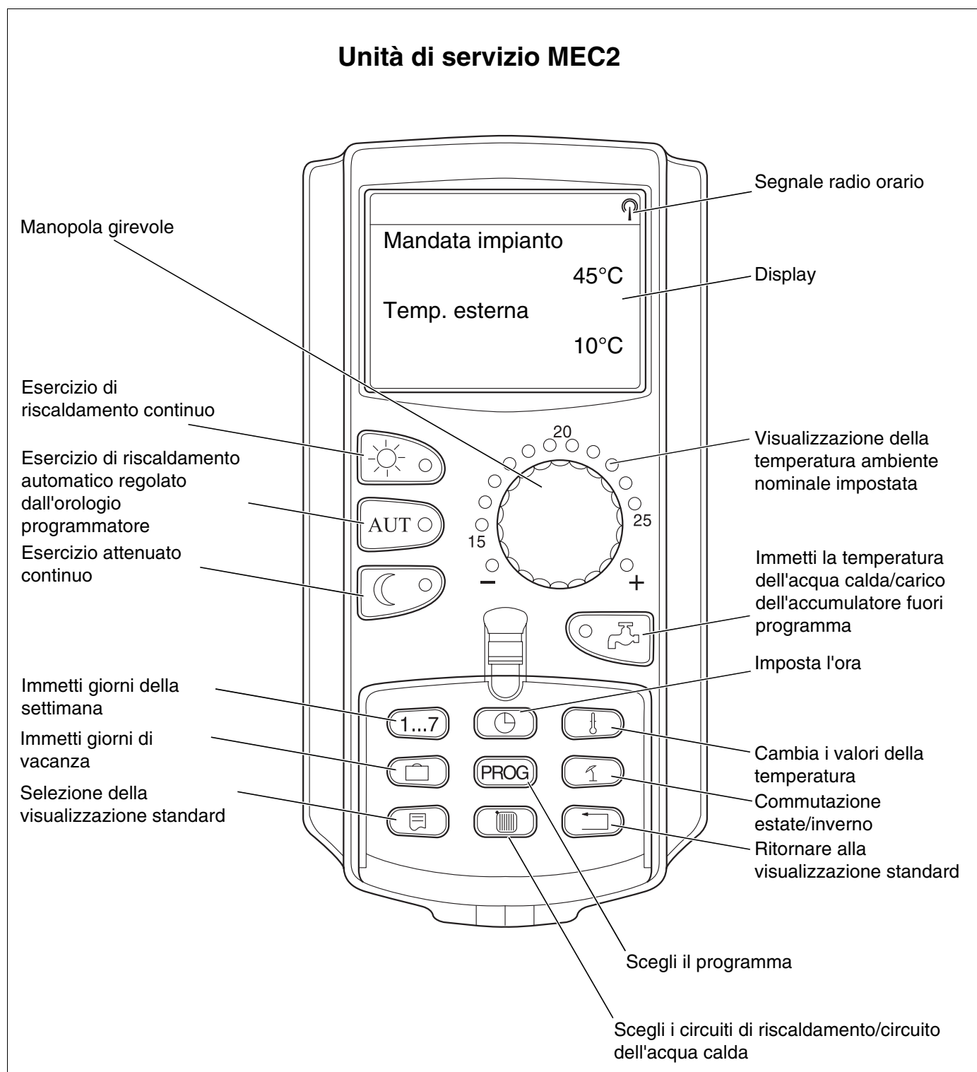
Fig. 5 Unità di servizio MEC2
