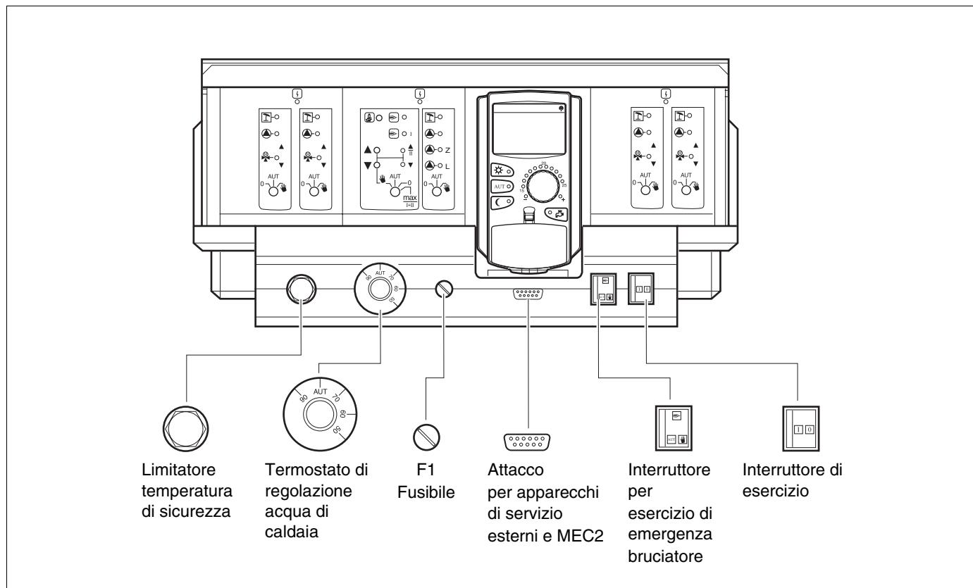
Fig. 1 Elementi di comando
