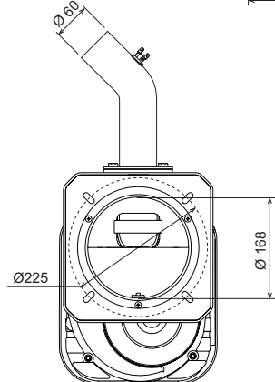
fig. 15 - Dimensionale SUN P12
