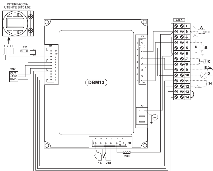
fig. 18 - Schema elettrico con morsettiera 14 poli
