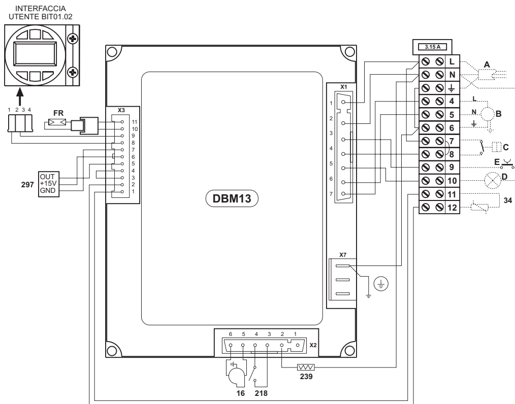
fig. 17 - Schema elettrico con morsettiera 12 poli
