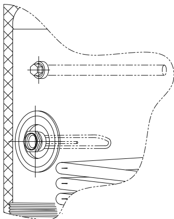
Fig. 8.1: Anodo resistenza flangiata
