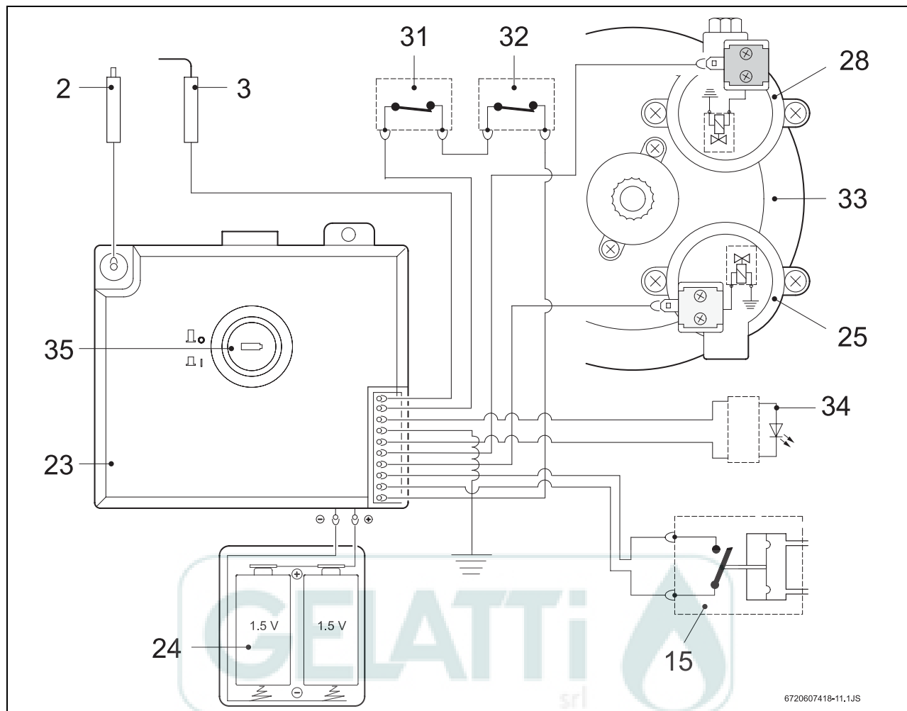
Fig. 3 Schema elettrico
