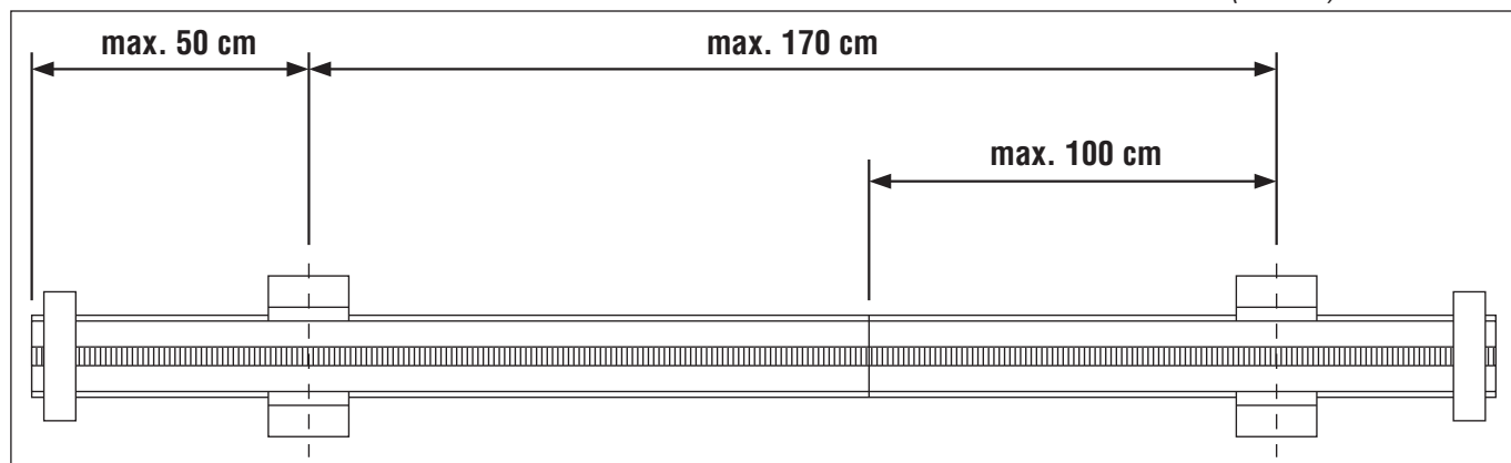
Distanze massime consentite tra le basi dei binari
