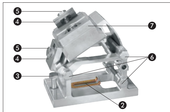
Supporto del binario per tagli su scale
