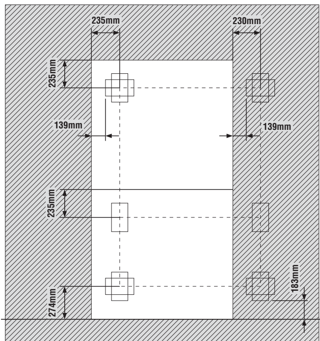
Distanze tra i tasselli
