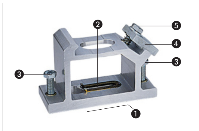
Supporto del binario per tagli normali
