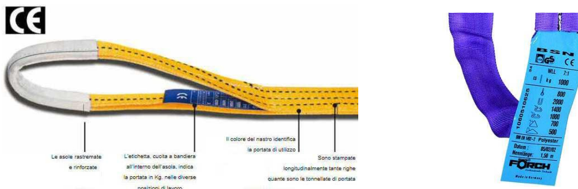
Nastri di sollevamento e certificazione CE
