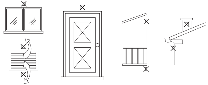
fig. 21 - Posizionamento sconsigliato sonda esterna
