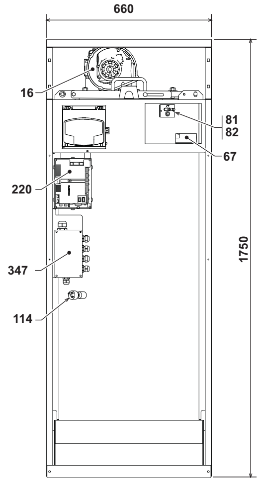
fig. 35 - Vista anteriore modello 125
