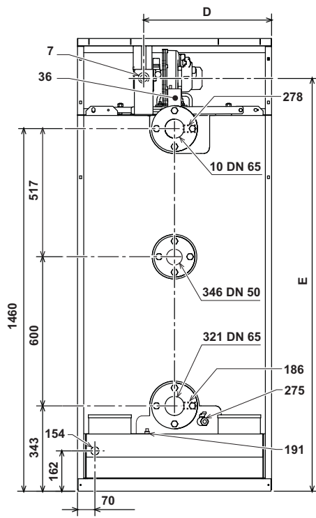
fig. 38 - Vista posteriore modelli 220/320
