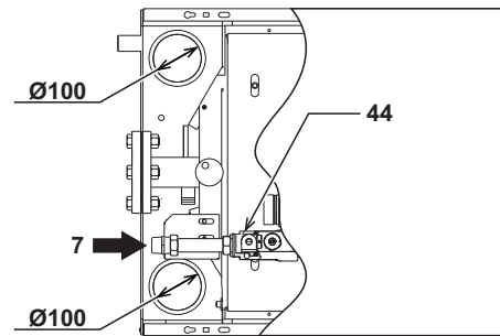
fig. 40 - Vista superiore modello 125
