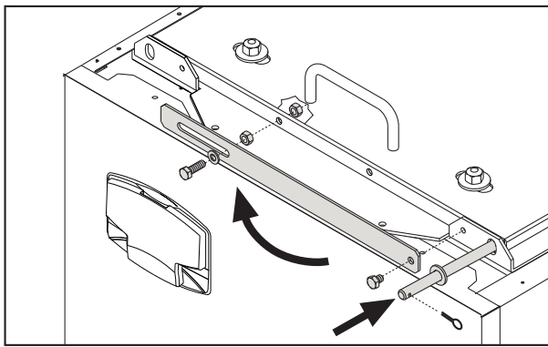
fig. 34 - Cambio lato apertura
