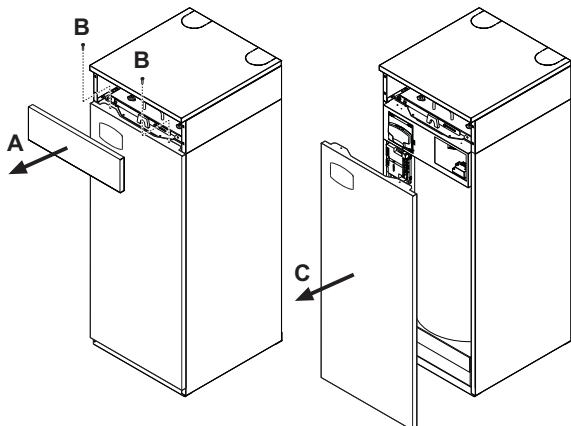
fig. 30 - Apertura del mantello
