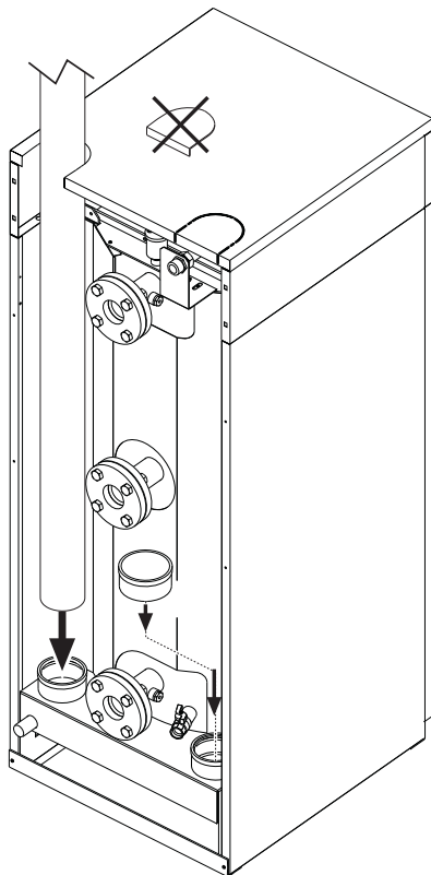
fig. 24 - Uscita fumi
