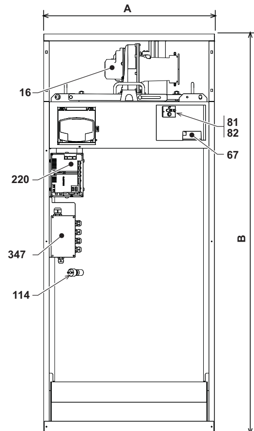
fig. 36 - Vista anteriore modelli 220/320
