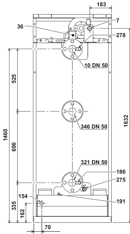
fig. 37 - Vista posteriore modello 125
