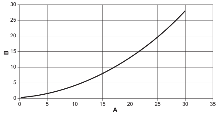
fig. 43 - Diagramma perdita di carico
