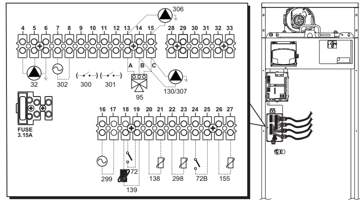
fig. 22 - Morsetteria elettrica
