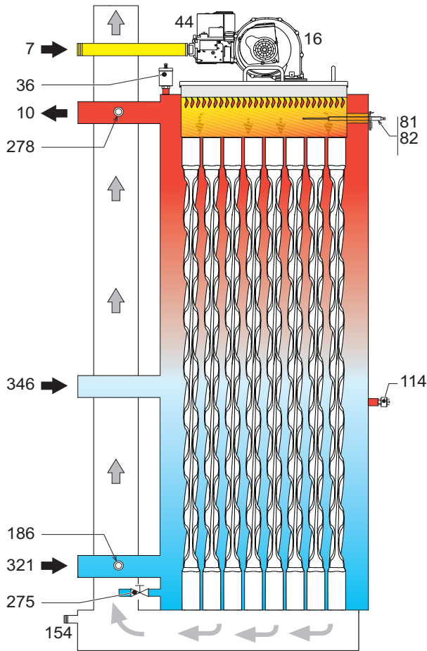
fig. 42 - Circuito idraulico
