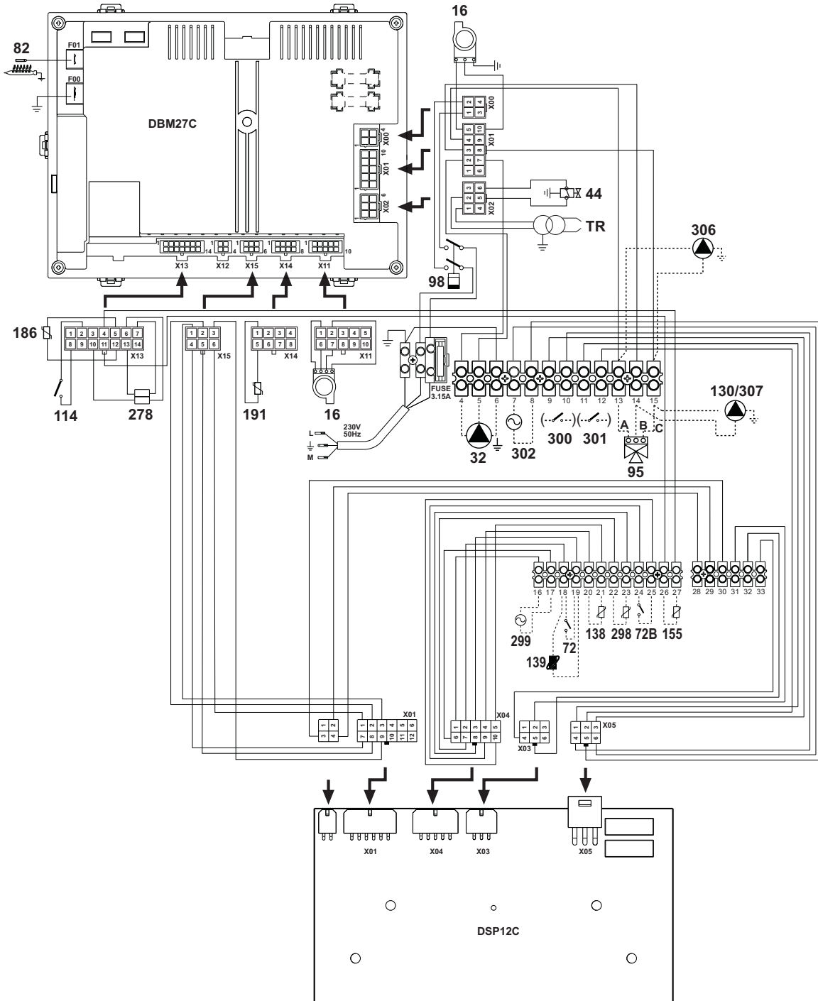
fig. 44 - Schema elettrico
