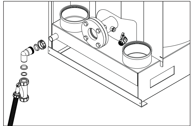
fig. 25 - Collegamento scarico condensa
