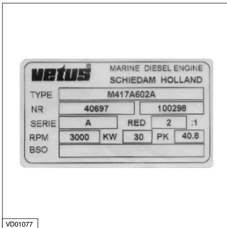
Targhetta di identificazione
