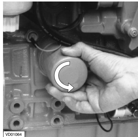
VD01064 Smontaggio del filtro dell'olio
