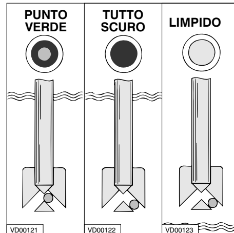
Funzionamento dell'idrometro
