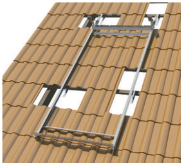
Installazione su superficie inclinata
