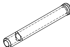
prolunga M-F coassiale ø80/125
