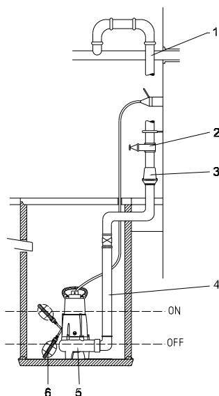
Figura 2 Esempio di installazione, vasca in calcestruzzo
