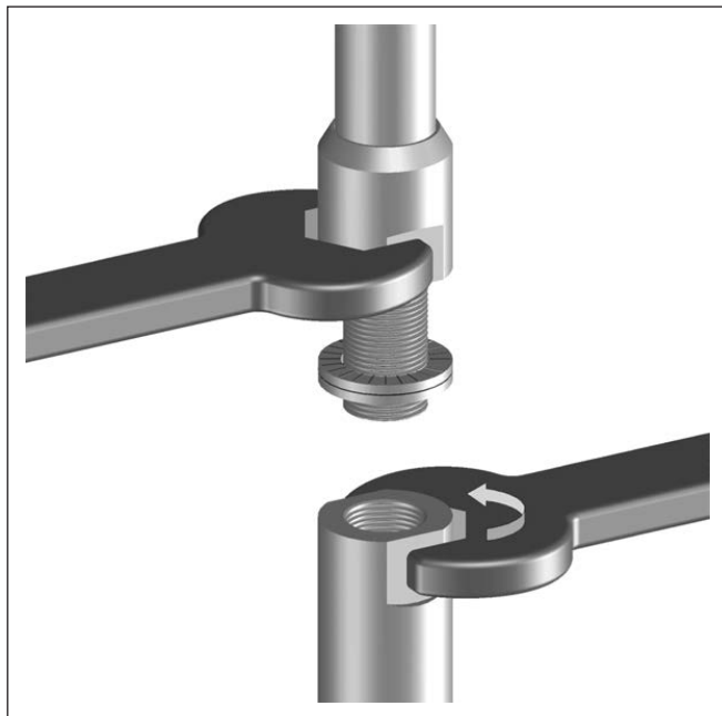
Figura 45: Sostituzione dello stilo ovv. della fune di misura
