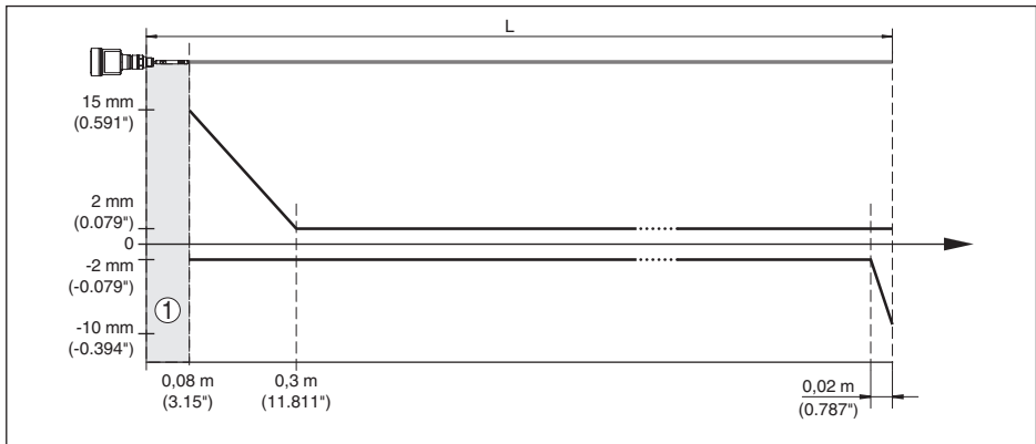
Figura 52: Scostamento di misura VEGAFLEX 82 in esecuzione a barra
