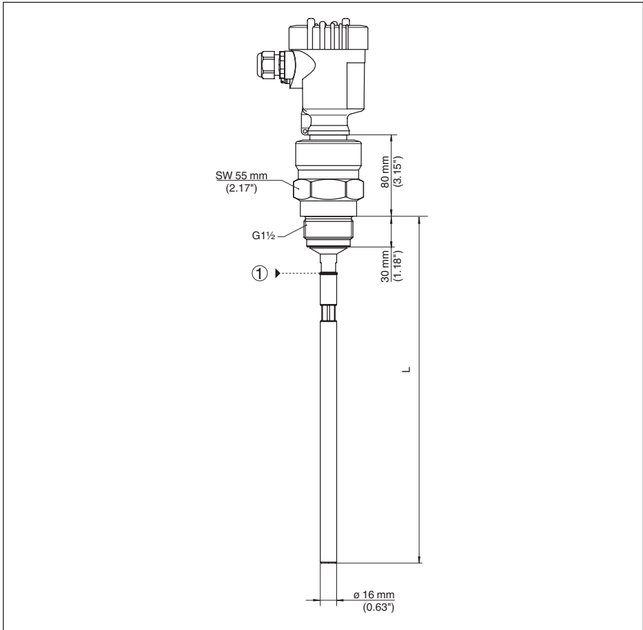
Figura 72: VEGAFLEX 82, stilo \varnothing 16 mm (0.63 in), esecuzione filettata
