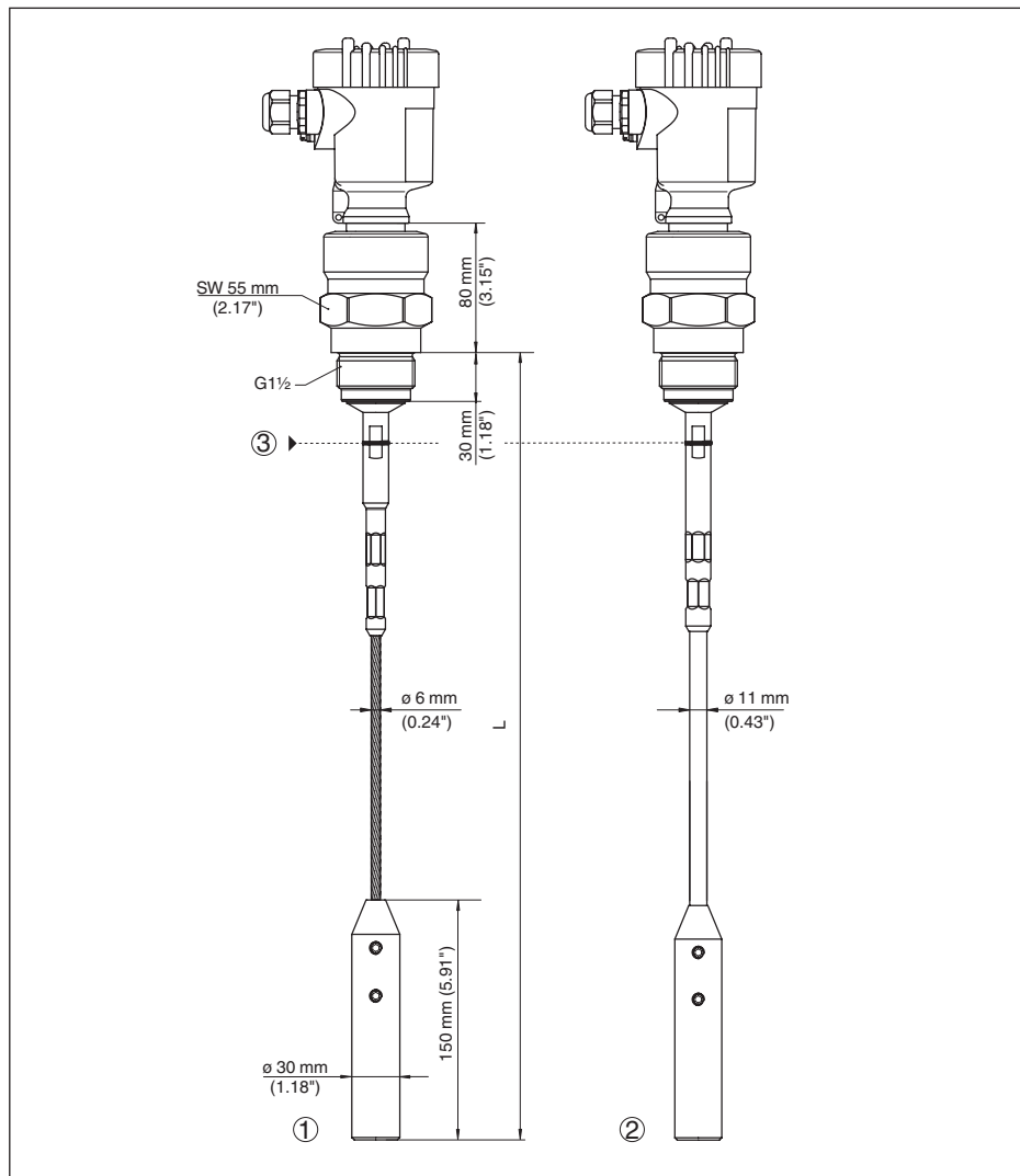
Figura 71: VEGAFLEX 82, fune \varnothing 6 mm (0.236 in)/ \varnothing 11 mm (0.433 in) esecuzione filettata con peso tenditore (tutti i pesi tenditori sono muniti di filettatura M12 per vite ad anello)
