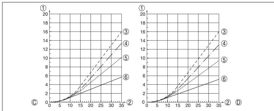
Figura 48: Massimo carico alla trazione per sabbia e cemento - fune: \varnothing 4 mm (0.157 in)
