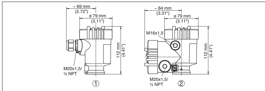
Figura 65: Custodie con grado di protezione IP 66/IP 67. Con tastierino di taratura con display incorporato l'altezza della custodia aumenta di 9 mm/0.35 in
