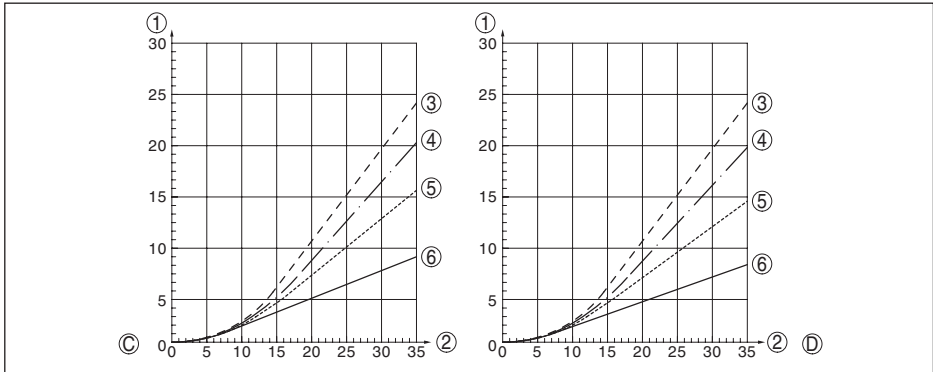
Figura 50: Massimo carico alla trazione per sabbia e cemento - fune: \varnothing 6 mm/ \varnothing 11 mm - con rivestimento in PA
