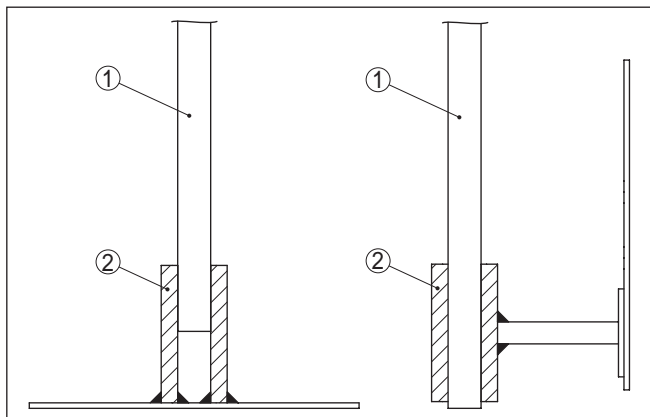
Figura 8: Fissaggio della sonda
