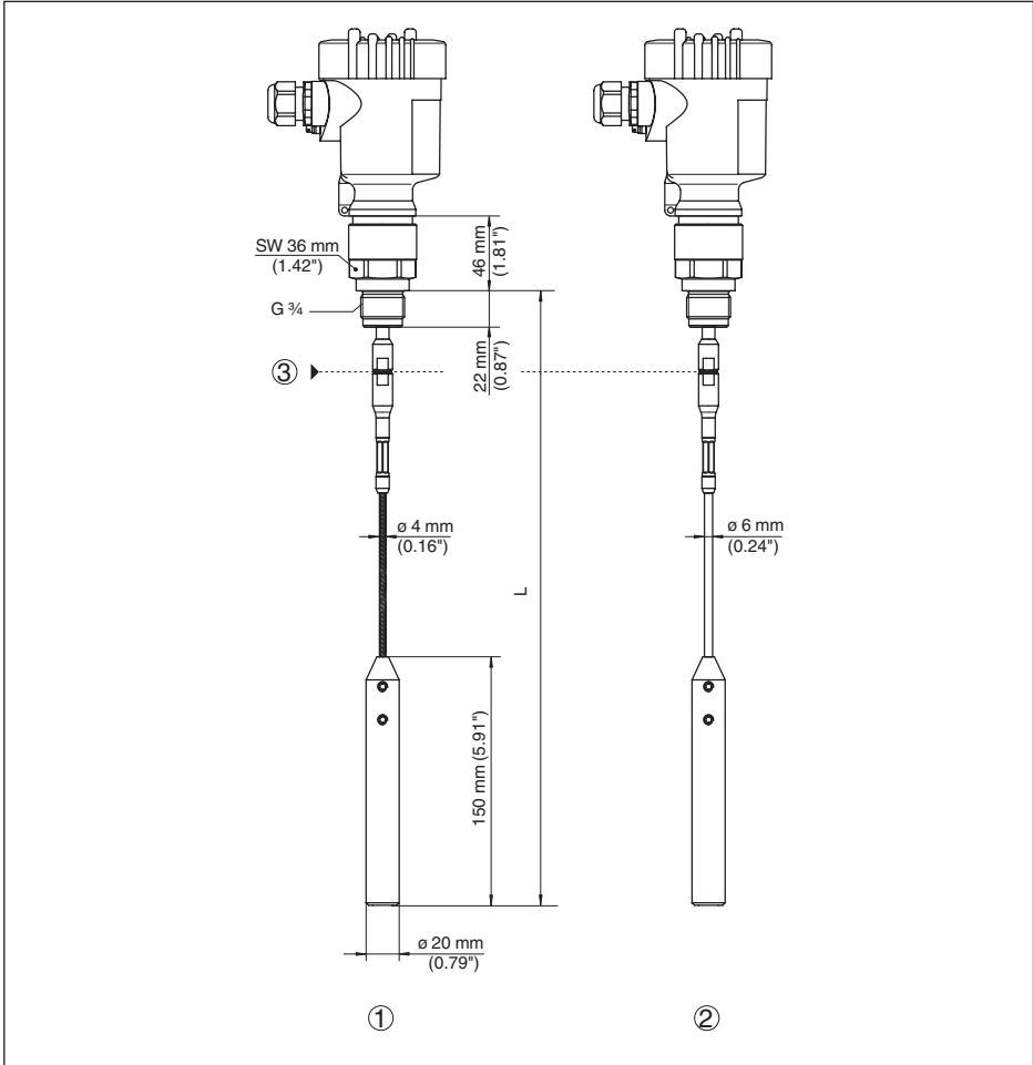
Figura 70: VEGAFLEX 82, fune \varnothing 4 mm (0.157 in)/ \varnothing 6 mm (0.236 in) esecuzione filettata con peso tenditore (tutti i pesi tenditori sono muniti di filettatura M12 per vite ad anello)
