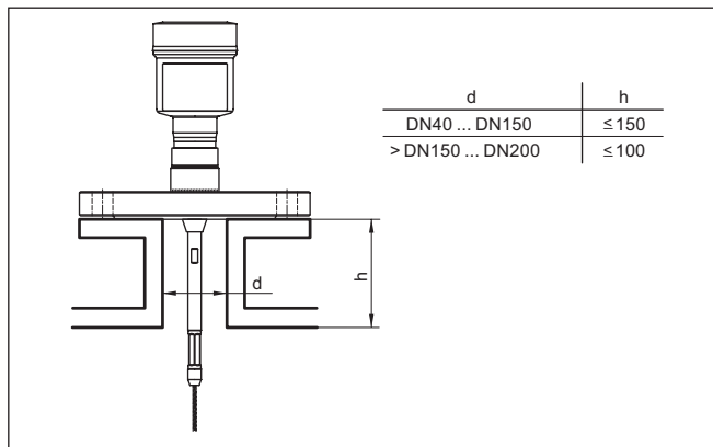
Figura 5: Tronchetto di montaggio
