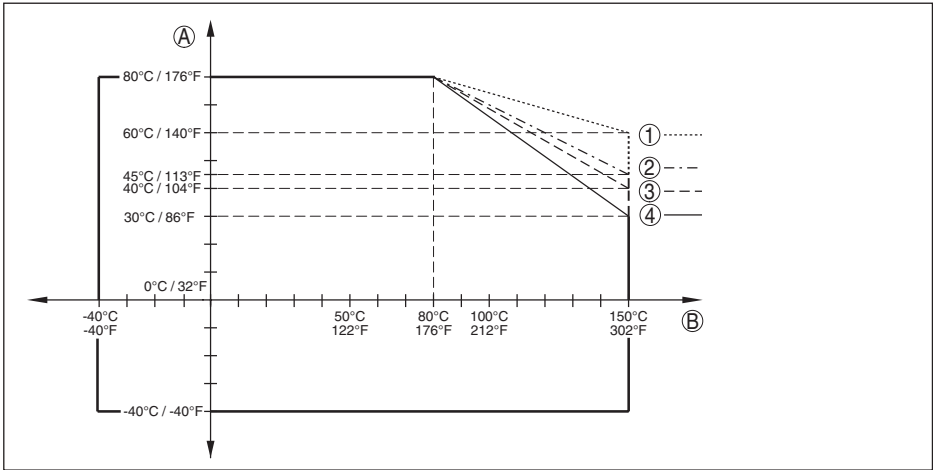
Figura 54: Temperatura ambiente - temperatura di processo, esecuzione standard
