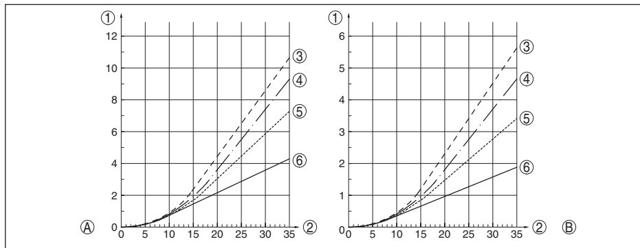
Figura 47: Massimo carico alla trazione per cereali e granulati plastici - fune: \varnothing 4 mm (0.157 in)
