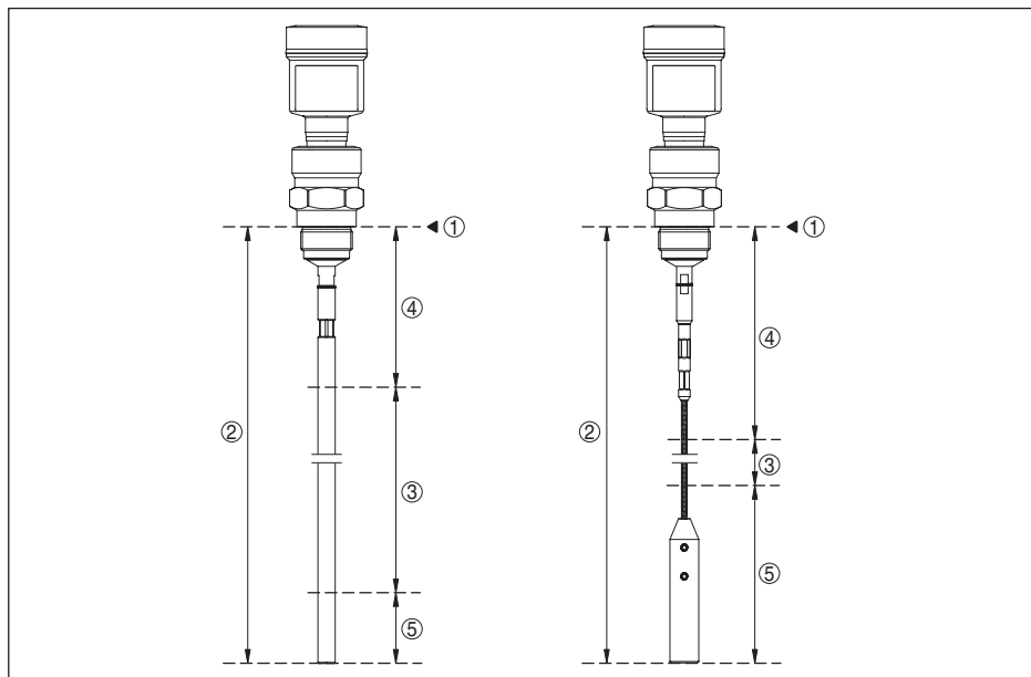
Figura 51: Campi di misura - VEGAFLEX 82
