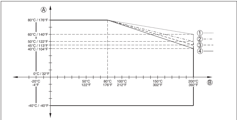
Figura 55: Temperatura ambiente - temperatura di processo, esecuzione con dissipatore termico
