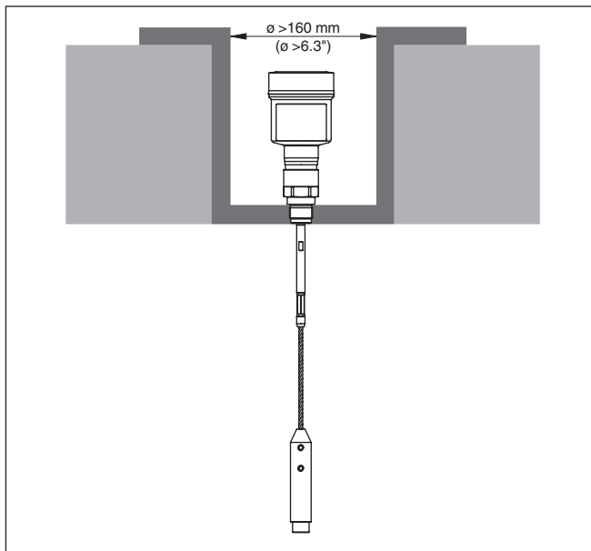
Figura 4: Montaggio in un silo di cemento
