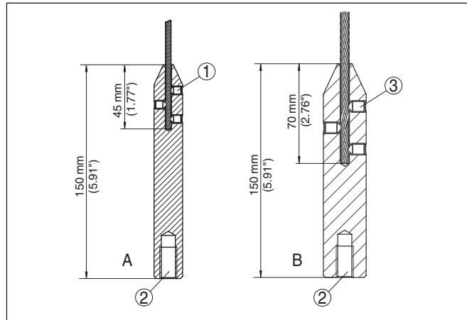
Figura 46: Riduzione della lunghezza della fune
