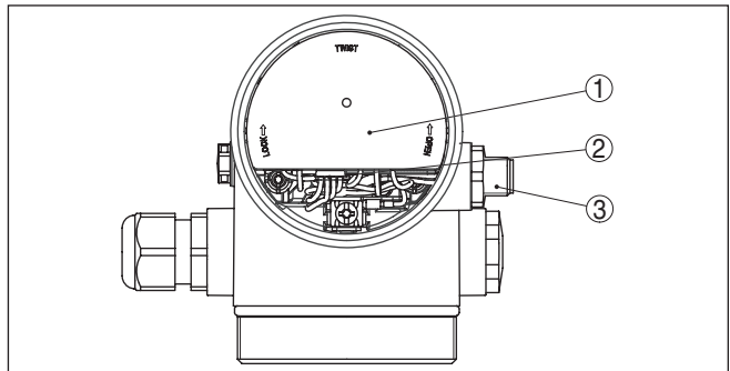
Figura 15: Vista sul vano dell'elettronica con DISADAPT per il collegamento dell'unità d'indicazione e di calibrazione esterna
