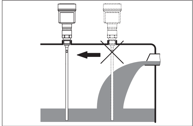
Figura 7: Montaggio del sensore in presenza del flusso di carico
