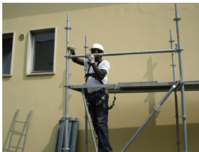
15) Montare il corrente inferiore
