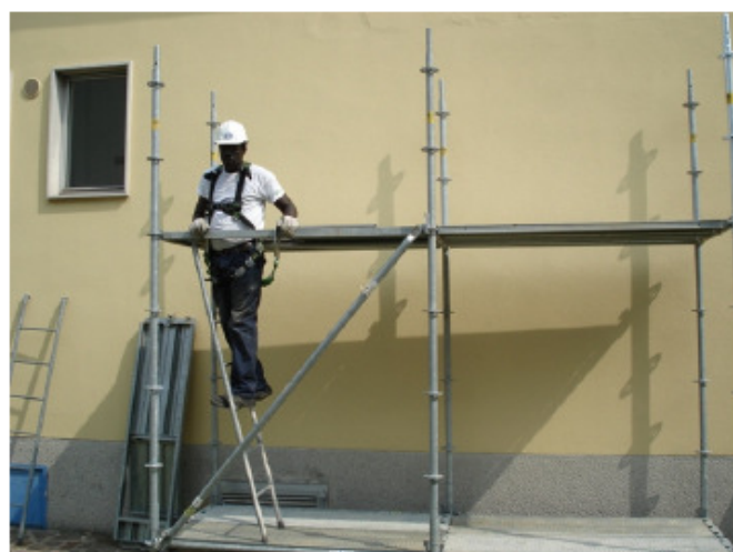
14) Assicurarsi alla tavola con botola, salire al piano superiore
