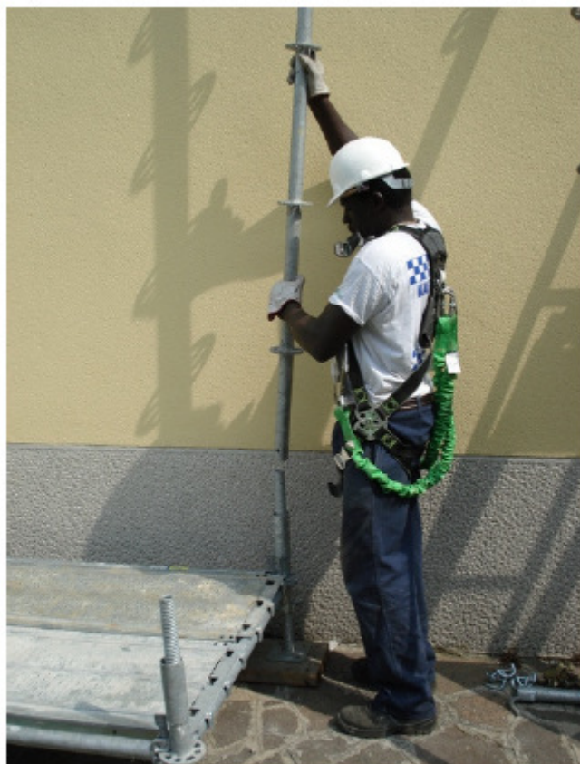
7) Infilare i montanti (da 3 metri al piano terra)
