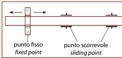
Fig. 18 Fissaggio delle tubazioni: tubo diritto, solo un punto fisso: corretto Pipe fixing: straight pipe, only one fixed point: suitable
