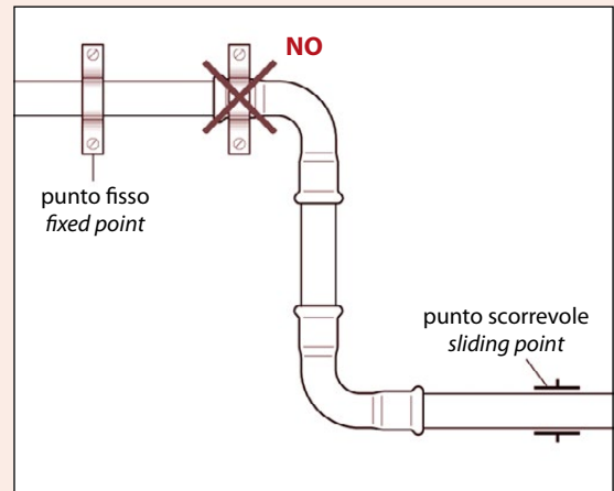
Fig. 20 Fissaggio delle tubazioni: punto fisso in corrispondenza del raccordo: errato Pipe fixing: fixed point on fitting: wrong
