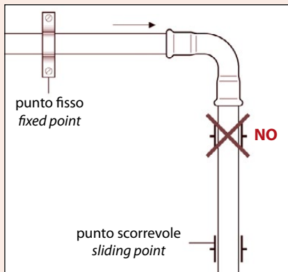
Fig. 19 Fissaggio delle tubazioni: punto scorrevole vicino al raccordo: errato Pipe fixing: sliding point near to fitting: wrong
