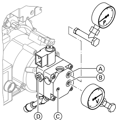
Pompa gasolio di produzione Danfoss, tipo BFP 31
