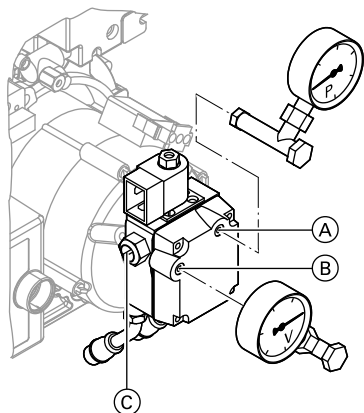
Pompa gasolio di produzione Danfoss, tipo BFP 31
