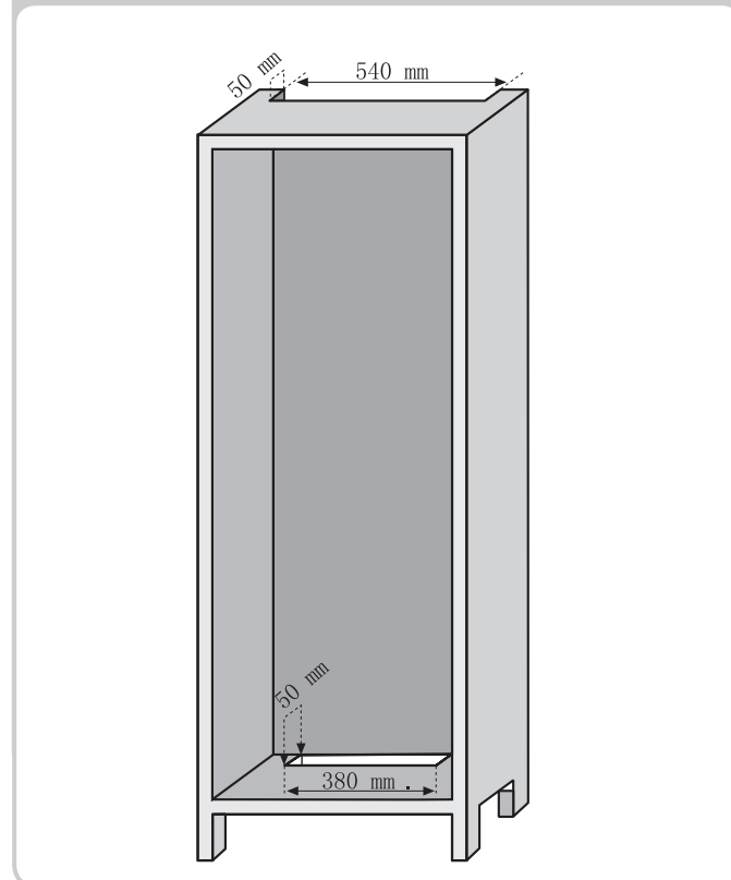
Distanza da mantenere tra la colonna e il soffitto
