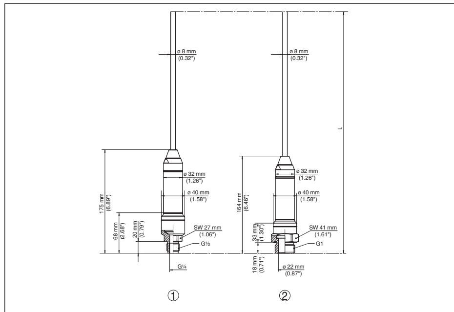
Figura 36: VEGABAR 86, esecuzione filettata
