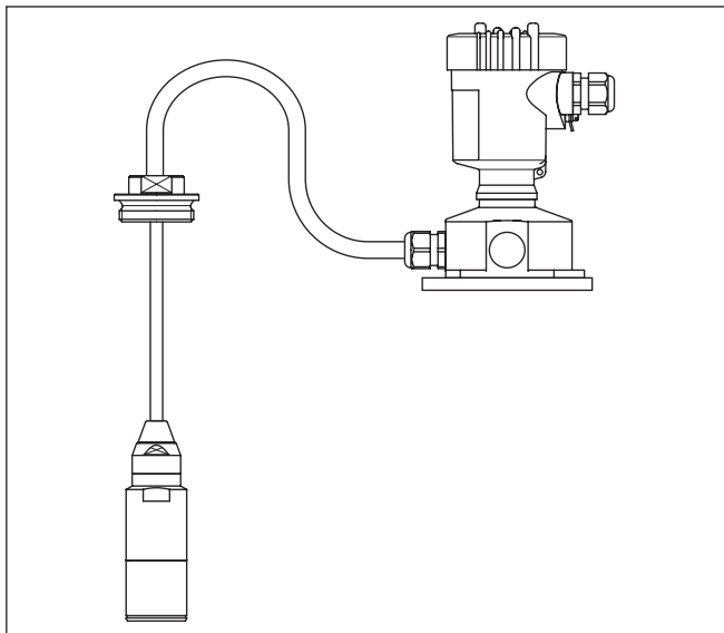
Figura 14: VEGABAR 86 in esecuzione IP 68 25 bar, non Ex e uscita del cavo assiale, custodia separata
