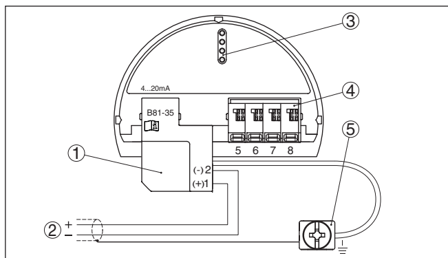
Figura 18: Vano dell'elettronica e di connessione custodia a una camera, vano di connessione custodia a due camere
