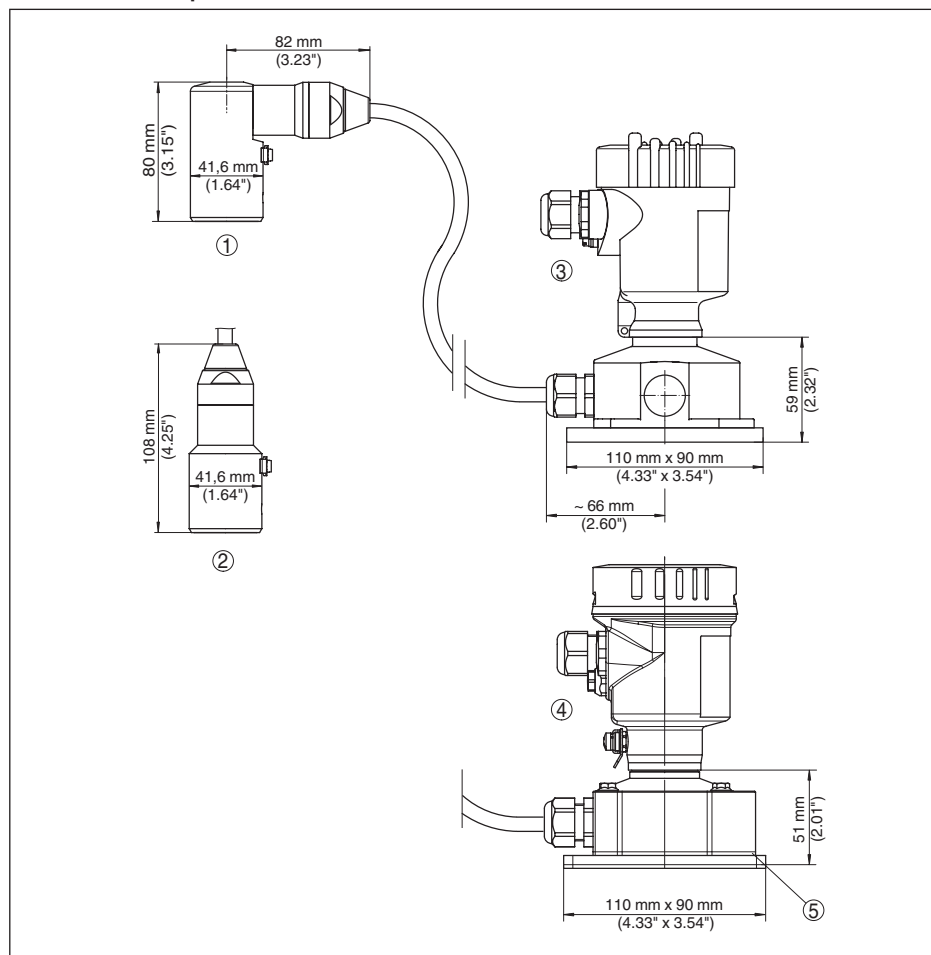
Figura 30: VEGABAR 86, esecuzione IP 68 con custodia esterna
