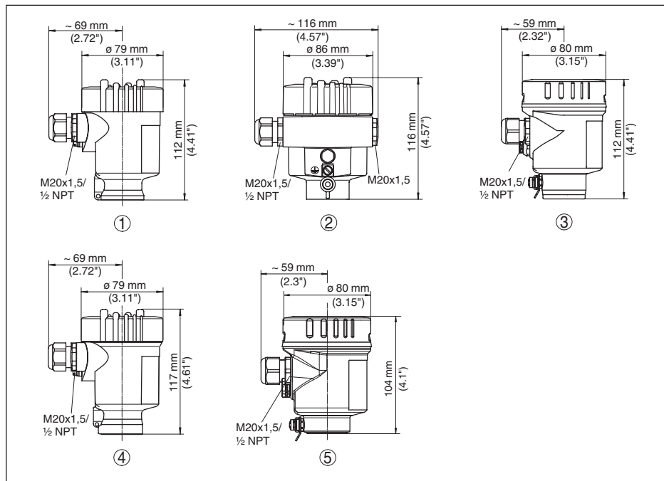
Figura 29: Esecuzioni della custodia con grado di protezione IP 66/67 e IP 66/68 (0,2 bar)
