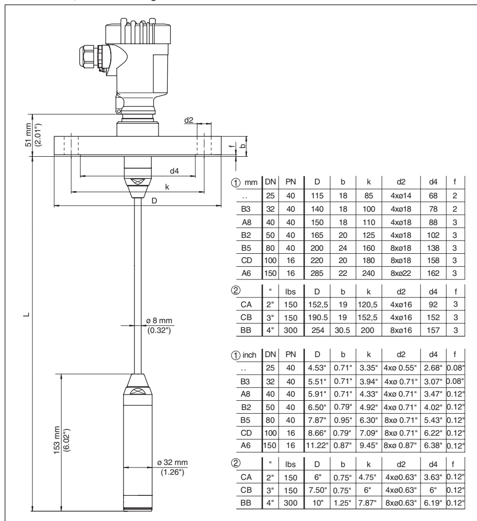
Figura 34: VEGABAR 86, attacco a flangia (esempio rilevatore del valore di misura 32 mm)
