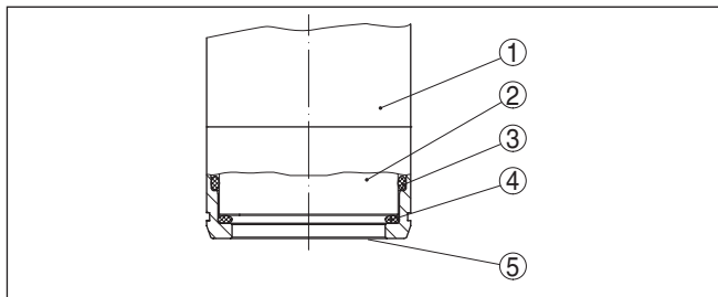
Figura 3: Montaggio affacciato della cella di misura in ceramica con doppia guarnizione
