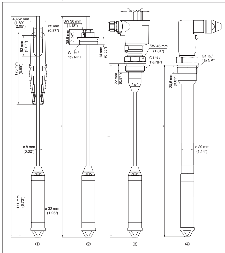
Figura 32: VEGABAR 86, elemento primario di misura 32 mm
