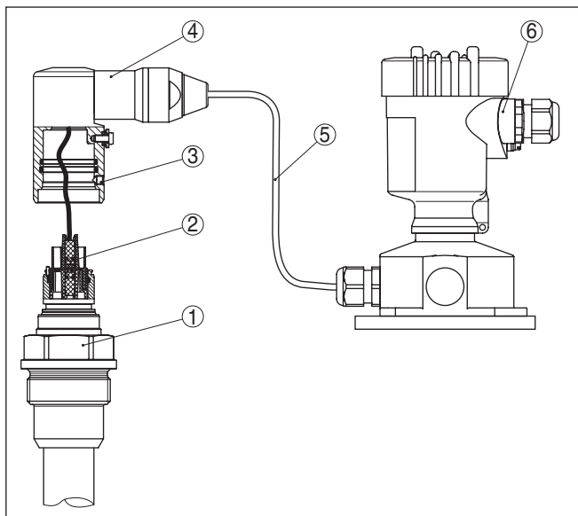
Figura 24: VEGABAR 86 in esecuzione IP 68 25 bar e uscita del cavo laterale, custodia esterna
