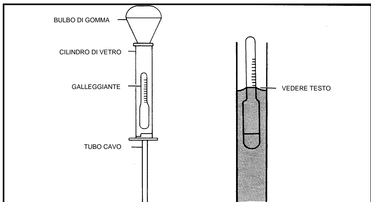
FIGURA 9 USO DELL'IDROMETRO
