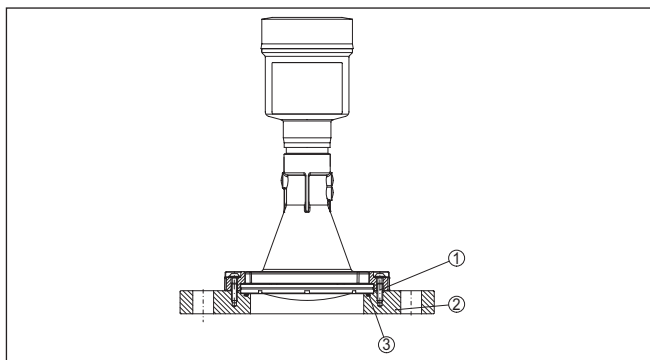
Figura 7: Flangia d'adattamento
