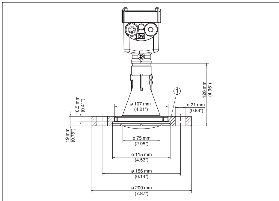
Figura 68: Sensore radar con flangia di raccordo
