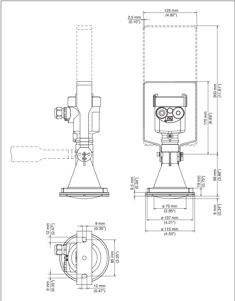
Figura 72: VEGAPULS 69, antenna a cono in resina, staffa di montaggio in lunghezza 170 o 300 mm
