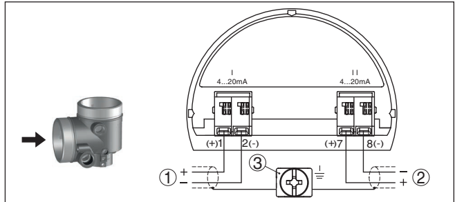
Figura 31: Vano di connessione custodia a due camere, elettronica supplementare - uscita in corrente supplementare
