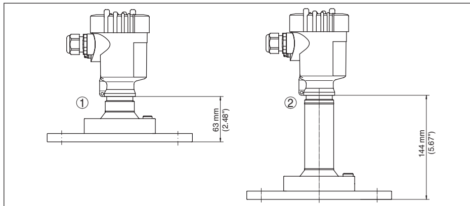
Figura 73: VEGAPULS 69, antenna a lente con profilo in metallo
