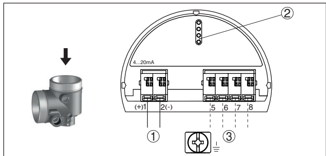
Figura 35: Vano dell'elettronica custodia a due camere Ex d ia
