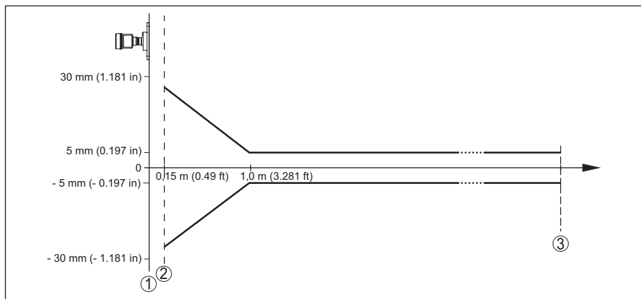
Figura 59: Scostamento di misura sotto condizioni di riferimento
