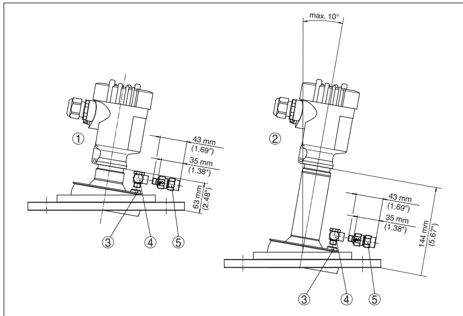
Figura 76: VEGAPULS 69, antenna a lente con profilo in metallo con supporto orientabile e attacco per spurgo
