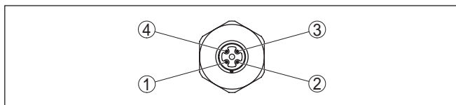
Figura 37: Vista del connettore a spina
