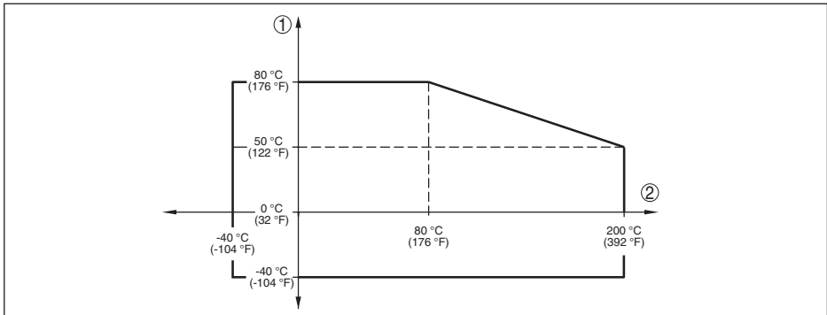
Figura 60: Temperatura ambiente - temperatura di processo, antenna a lente rivestita di metallo fino a +200 °C (392 °F)
