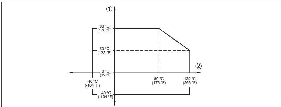
Figura 61: Temperatura ambiente - temperatura di processo, antenna a lente rivestita di metallo fino a +130 °C (266 °F)
