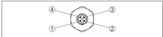
Figura 39: Vista sul connettore a spina M12 x 1
