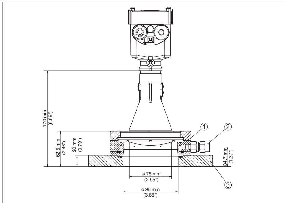
Figura 71: VEGAPULS 69, flangia di adattamento e attacco per spurgo
