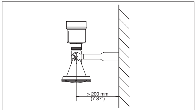
Figura 4: Montaggio a parete orizzontale tramite la staffa di montaggio lunga 170 mm
