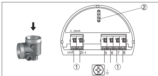
Figura 29: Vano dell'elettronica con custodia a due camere
