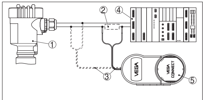
Figura 46: Collegamento del PC via HART alla linea del segnale
