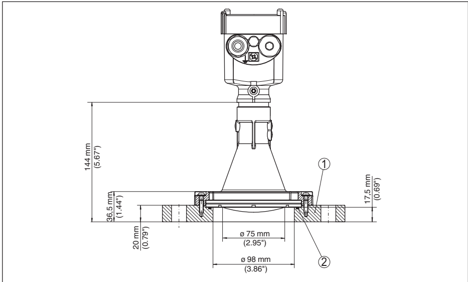
Figura 70: Sensore radar con flangia di adattamento
