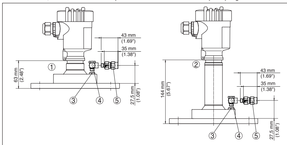
Figura 74: VEGAPULS 69, antenna a lente con profilo in metallo con attacco per spurgo
