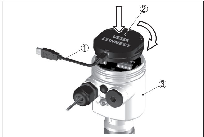
Figura 45: Collegamento diretto del PC al sensore via adattatore d'interfaccia
