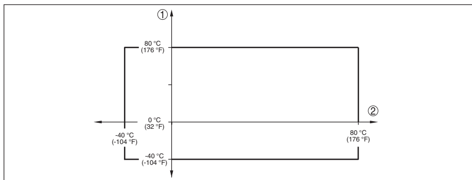
Figura 62: Temperatura ambiente - temperatura di processo, antenna a cono in resina
