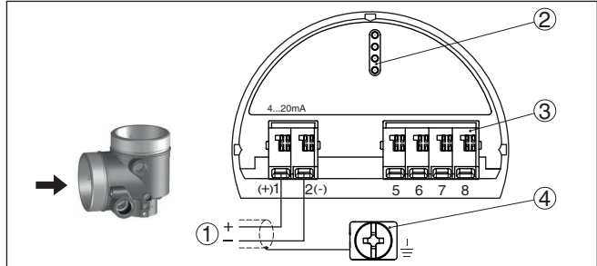
Figura 34: Vano di allacciamento custodia a due camere
