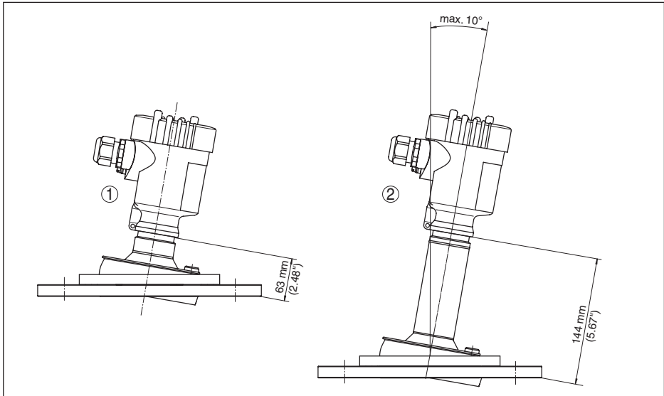
Figura 75: VEGAPULS 69, antenna a lente con profilo in metallo e supporto orientabile
