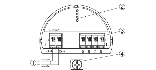
Figura 28: Vano dell'elettronica e di connessione della custodia ad una camera
