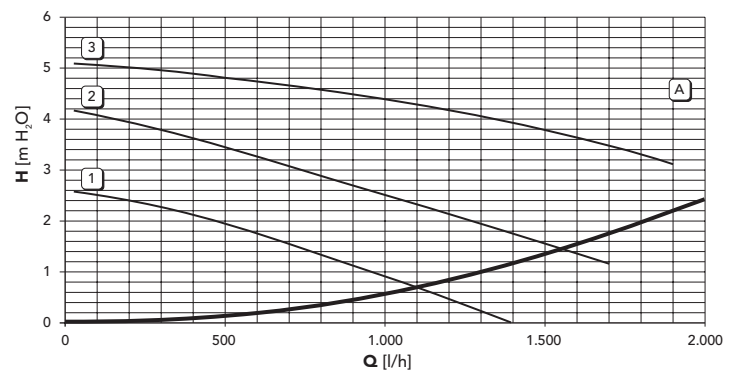
fig. 22 - Perdita di carico / prevalenza circolatore
