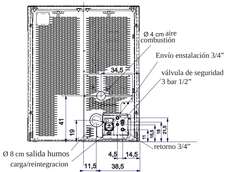
VUELTA
