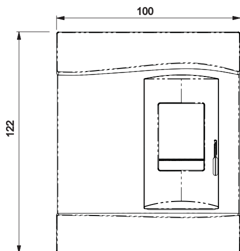
FRONTE
