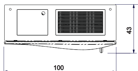
PLANTA
