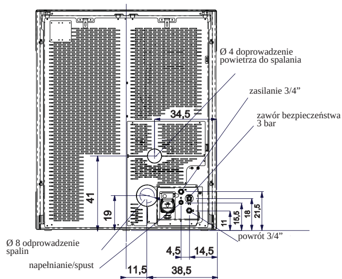
TYŁ
