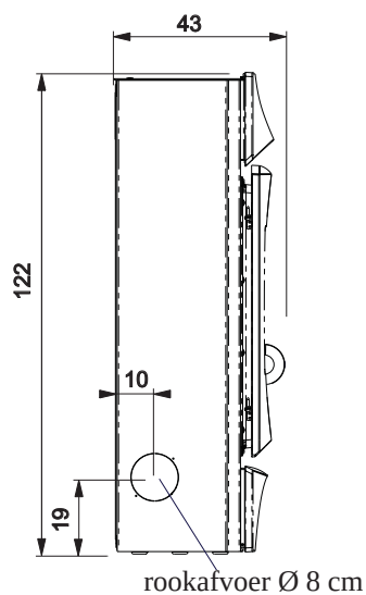
KANT
