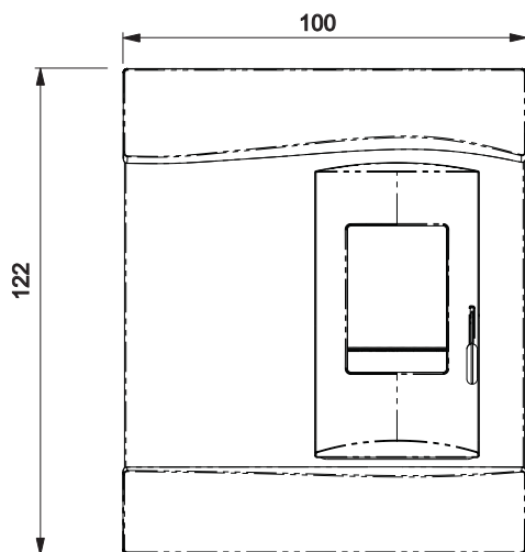
FRENTE
