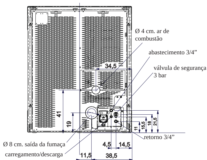
ATRÁS
