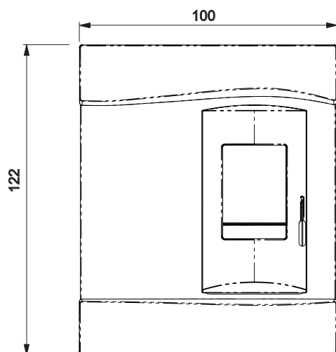
PRZÓD
