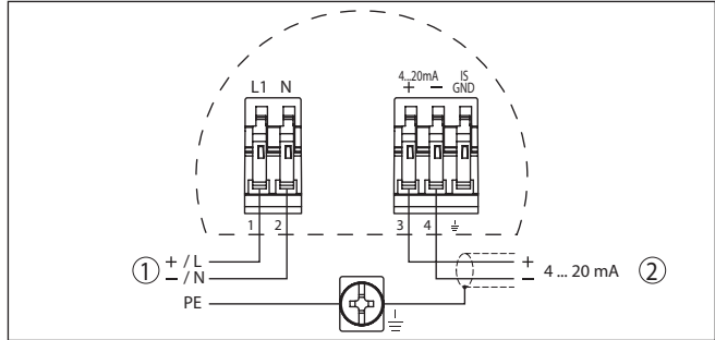
Figura 11: Schema di allacciamento custodia a due camere
