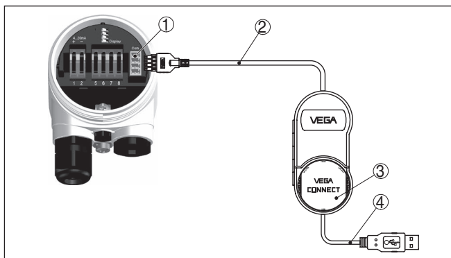
Figura 16: Collegamento via VEGACONNECT esterno
