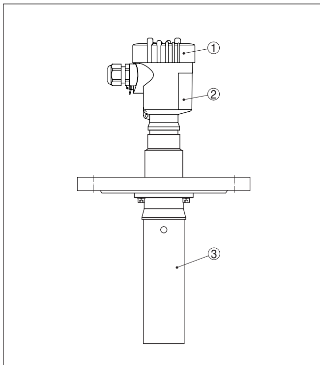
Figura 1: VEGAPULS 66 in esecuzione a flangia fino a 150 °C con custodia di resina
