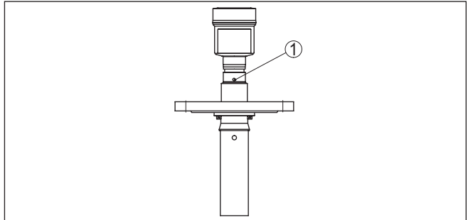
Figura 4: Posizione del piano di polarizzazione del VEGAPULS 66
