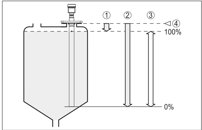
Figura 3: Campo di misura (campo di lavoro) e massima distanza di misura
