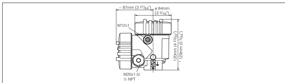
Figura 20: Custodia a due camere di alluminio e/o di acciaio speciale (con tastierino di taratura con display incorporato, l'altezza della custodia aumenta di 9 mm/0.35 in)
