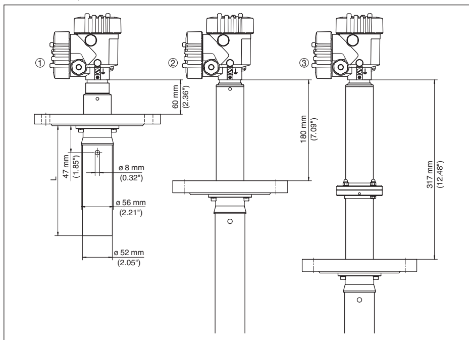
Figura 21: VEGAPULS 66, esecuzione con tubo di livello 15)
