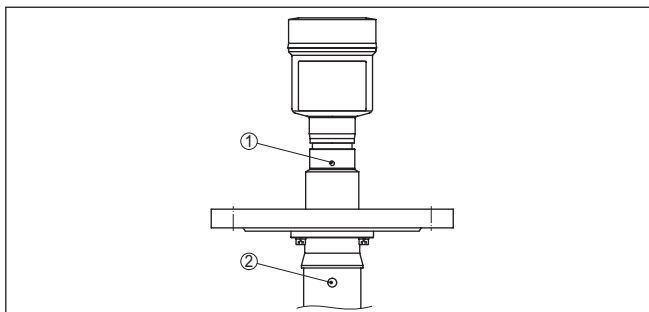
Figura 5: Contrassegno di polarizzazione
