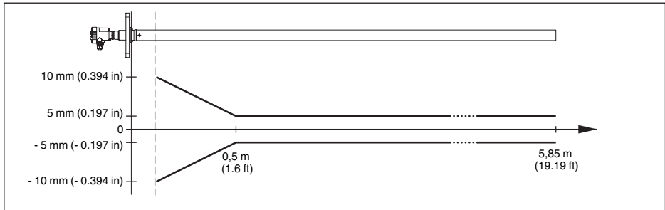
Figura 19: Scostamento di misura VEGAPULS 66 con tubo di livello
